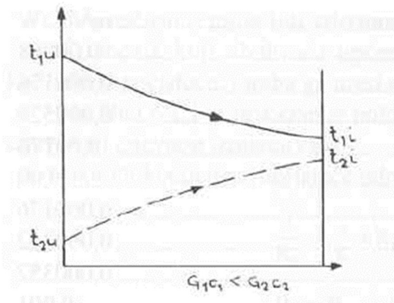
Slika 15. Dijagram za istosmjerno strujanje [5]
