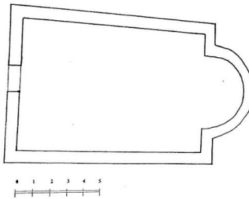
Slika 29. Tlocrt crkve sv. Duha
