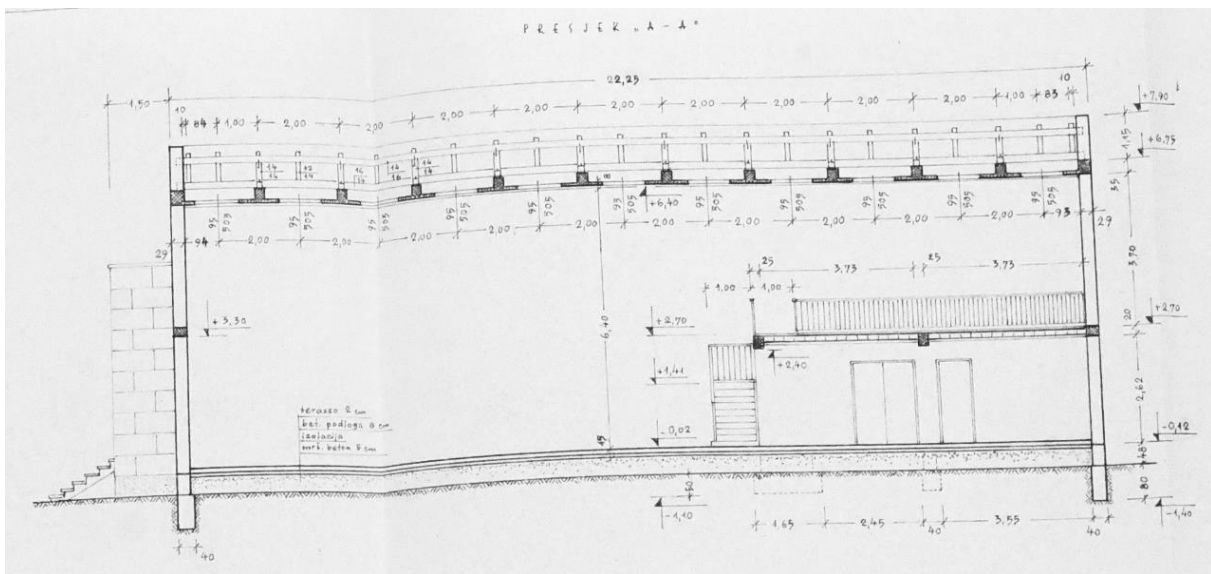
Slika 16 Presjek „A-A“ (dio sveukupnog nacrta projekta) (Izvor: Arhiva SGIMV)
