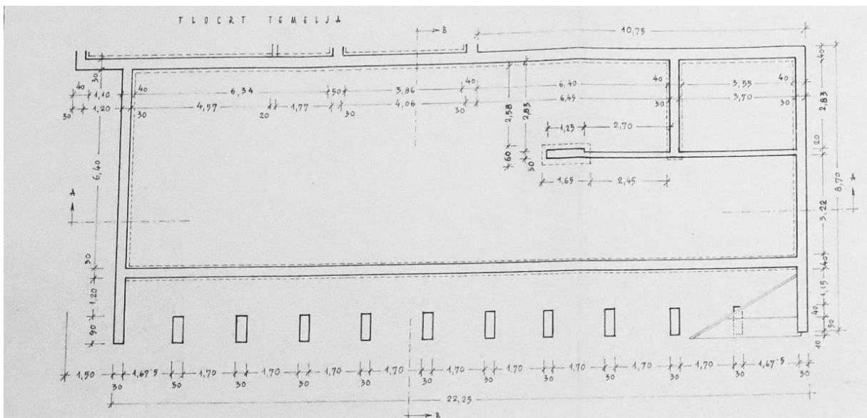
Slika 14 Tlocrt temelja Galerije (dio sveukupnog nacrt projekta) (Izvor: Arhiva SGIMV)
