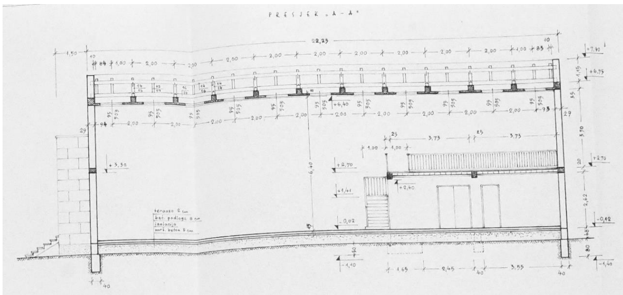
Slika 16 Presjek „A-A“ (dio sveukupnog nacrtu projekta) (Izvor: Arhiva SGIMV)
