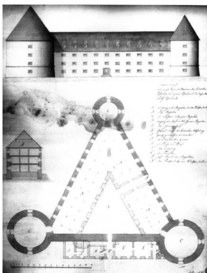
Slika 6: Nacr i tlocrt utvrde Sisak (S. SEKULIĆ-GVOZDANOVIĆ, 2019, 82.)
