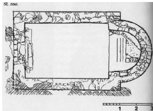
Slika 41: Tlocrt romaničke kapelice (Z: HORVAT, 2014, 174.)
