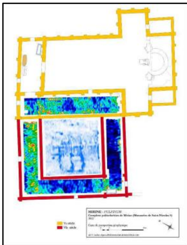
Slika 10: Tlocrtni plan bazilike u Mirinama (M. ČAUŠEVIĆ-BULLY, S. BULLY, 2016, 20.)
