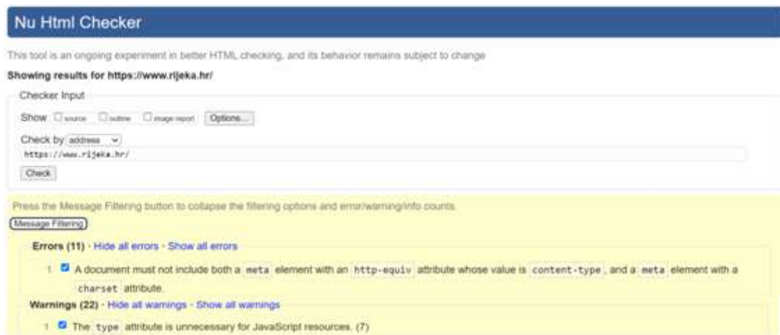
Slika 26. Rezultati analize W3C Validator (Rijeka)
