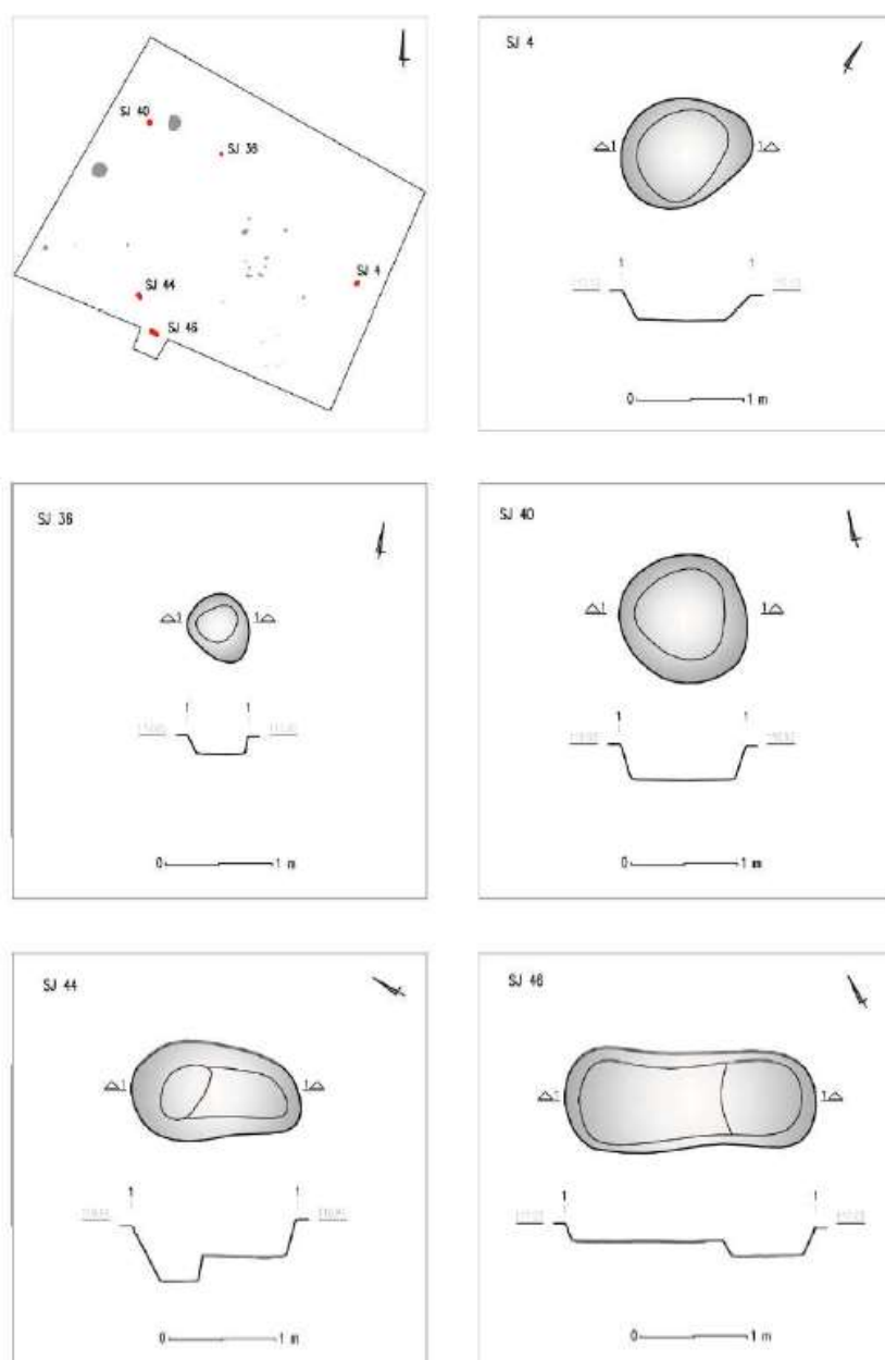
Slika 22. Položaj jama i njihovi oblici s lokaliteta Turbina 1 (M. DIZDAR, T. SEKELJ IVANČAN, 2017, 66.)
