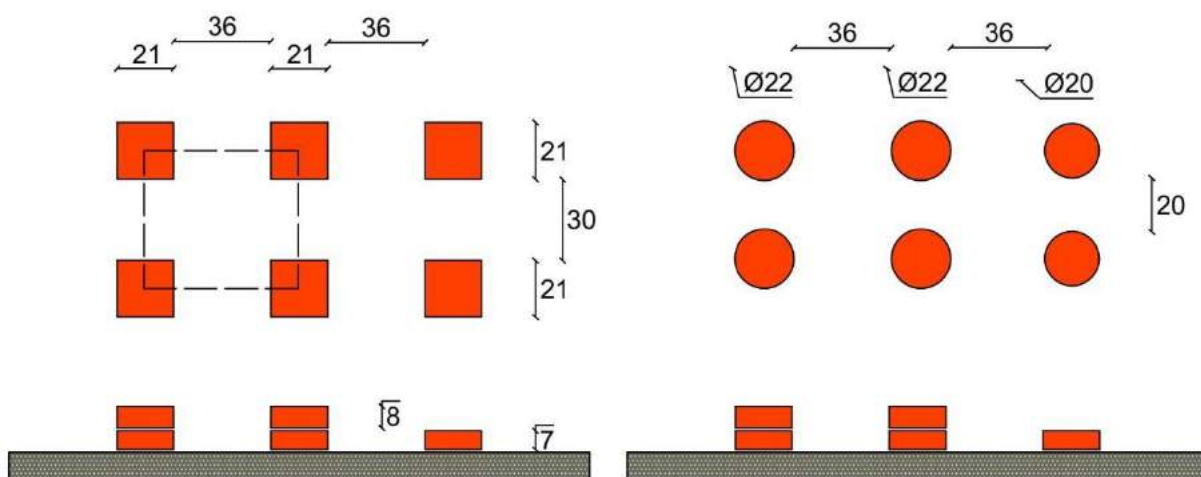
Slika 9. Pozicija i presjek suspenzura hipokausta iz Prostorije I i II. (Izradio M. Rašić prema originalu odgovornog arhitekta Ferhada Mulabegovića 1978. god.)
