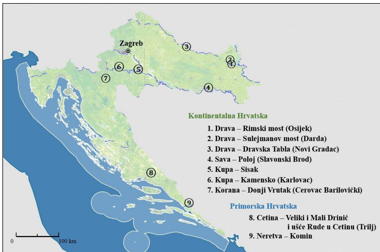
Slika 9. Prikaz najvažnijih spomenutih podvodnih arheoloških pozicija u hrvatskim rijekama (preuzeto s https://geoportal.dgu.hr/ , doradila: autorica).
