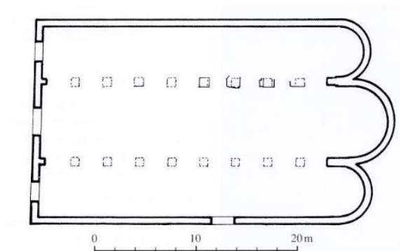
Slika 18: Tlocrt Sv. Marije Velike (T. MARASOVIĆ, 2008, 343)
