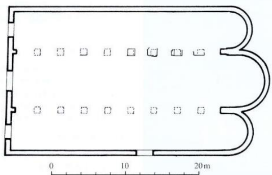
Slika 18: Tlocrt Sv. Marije Velike (T. MARASOVIĆ, 2008, 343)
