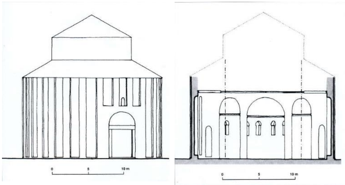
Slika 10: Pretpostavljeni vanjski izgled i presjek prvobitne rotonde (T. MARASOVIĆ, 2008, 307)
