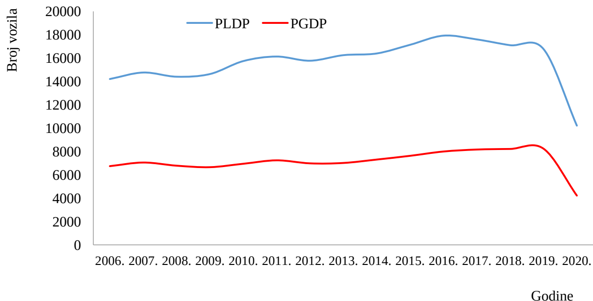
Slika 9. Prosječni godišnji i ljetni dnevni ljetni promet na prometnici A7 Rupa – Jurdani
