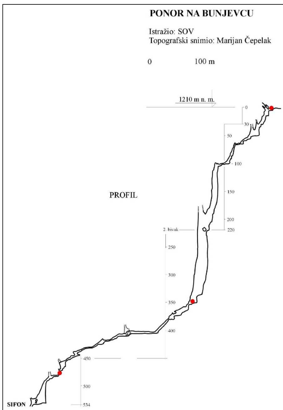
Slika 16. Speleološki nacrt Ponora na Bunovcu u NP Paklenica, primjer koljeniĉastog ili stubastog speleološkog objekta (Kuhta i dr., 2002)
