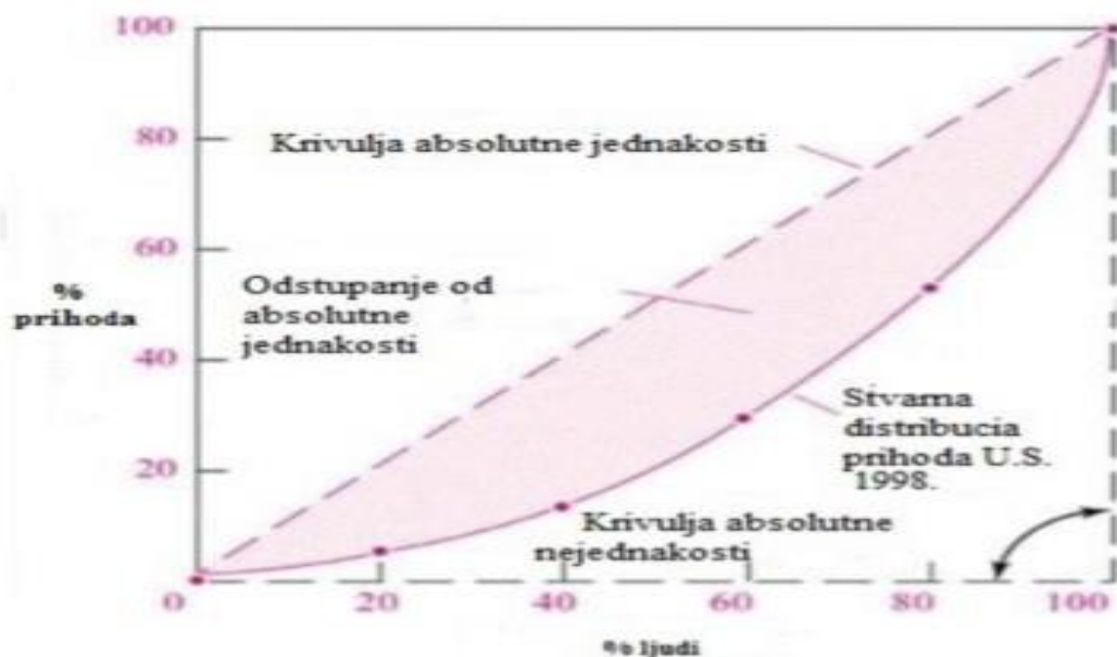
Slika 1- Lorenzova krivulja
