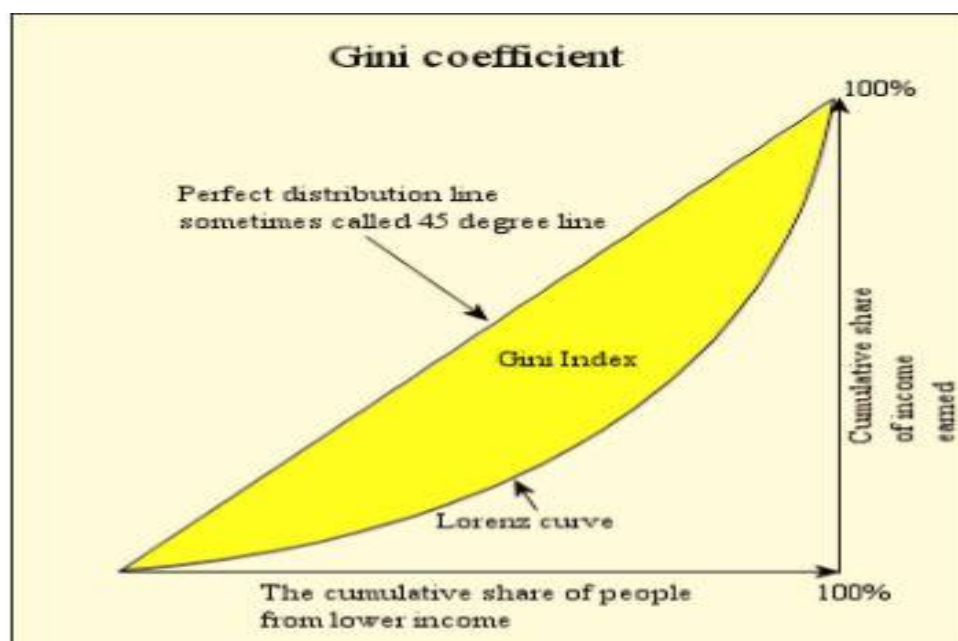
Slika 2- Ginijev koeficijent
