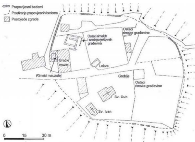
Slika 36. – Tlocrt škripske gradine (preuzeto od: STANČIĆ et al., 2004., 50.)
