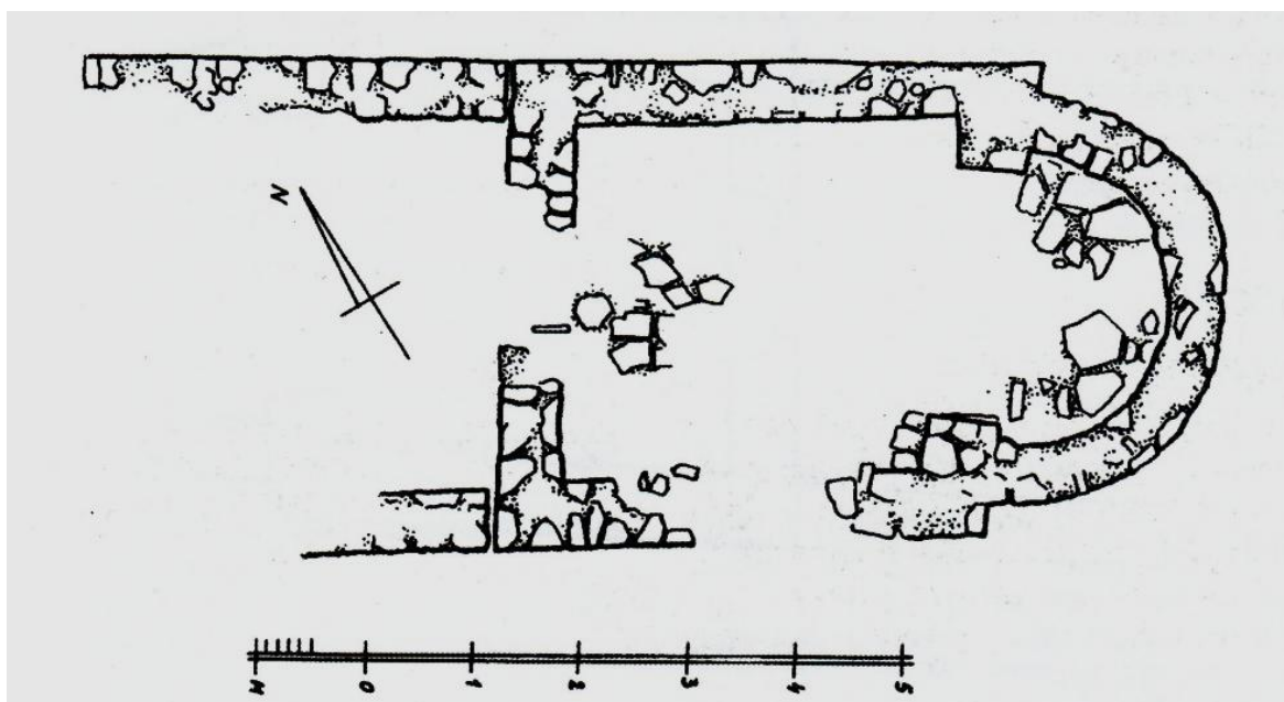
2. Tlocrt crkve Sv. Viktora na Citoriju kod mjesta Sali na Dugom otoku (I. Petricioli, 1987.)
