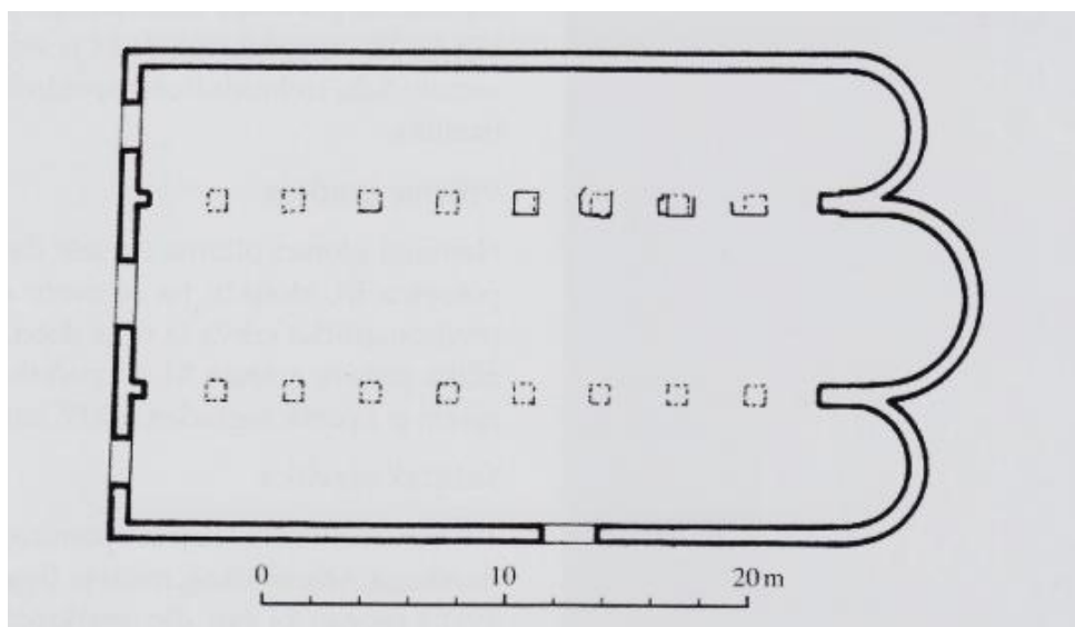
2. Zadar, Sv. Marija – tlocrt bazilike (P. Vežić, 1975.)
