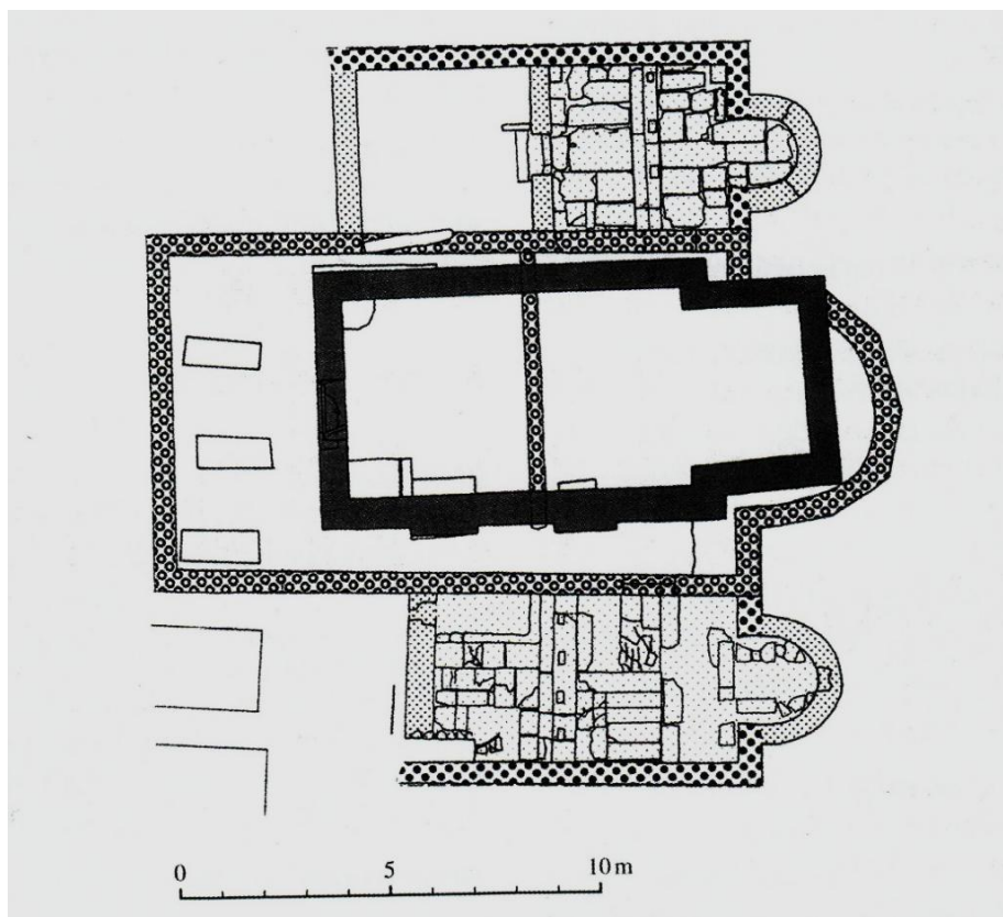
2. Lepuri, Sv. Martin – tlocrt crkve (N. Jakšić, 2000.)
