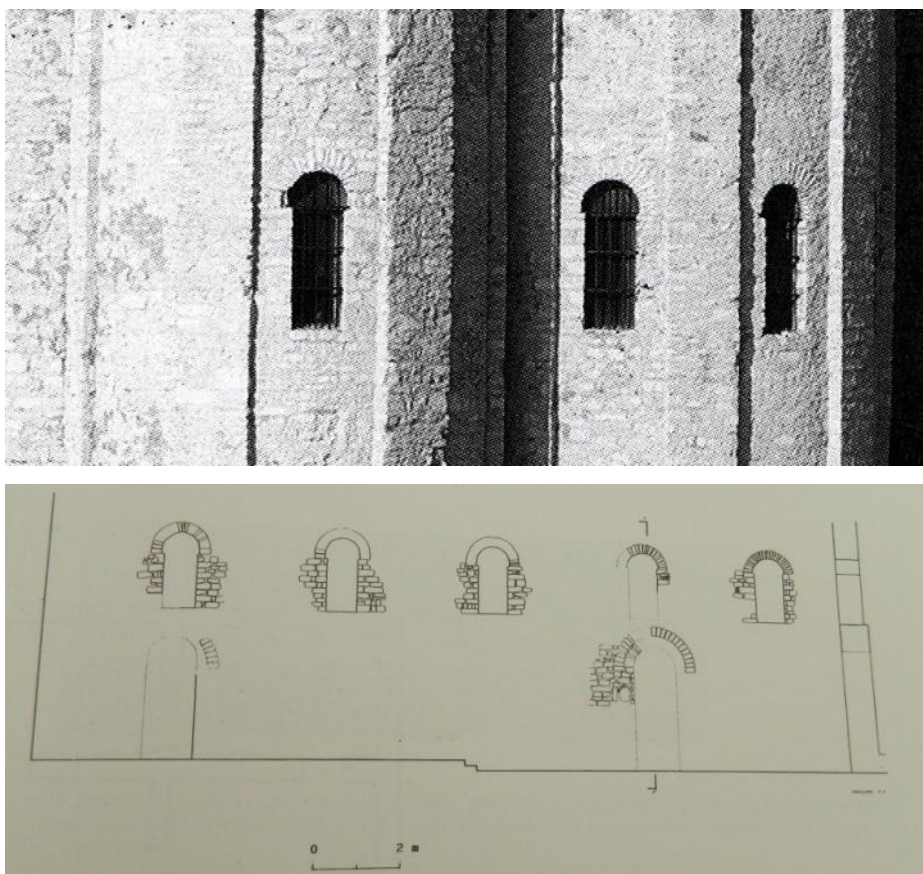
Sl. 29. Monofore na crkvi Sv. Donata (gore) i na južnom zidu župne crkve Sv. Asela u Ninu (dolje), (crtež rekonstrukcije prema: P. Vežić, 1996.)
