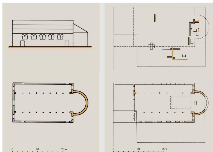
2. Zadar, Sv. Toma – tlocrt, grafička rekonstrukcija i definirani ostatci bazilike (P. Vežić, 2005.)
