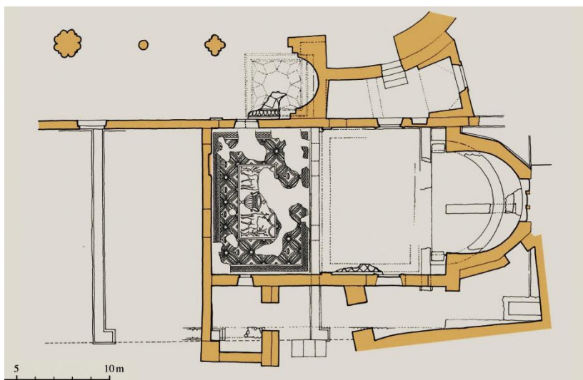
1. Zadar (Iader) – tlocrt sakristije katedralnog kompleksa (P. Vežić, 2005.)
