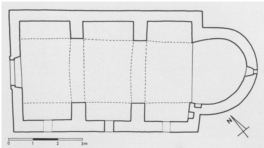
1. Vrgada, Sv. Andrija – tlocrt crkve (M. Domijan, 1983.)
