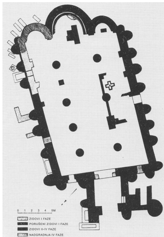
1. Biograd, Katedrala – tlocrt i razvojne faze crkve na položaju Glavica (L. Jelić; objavio: F. Buškariol, 1990.)
