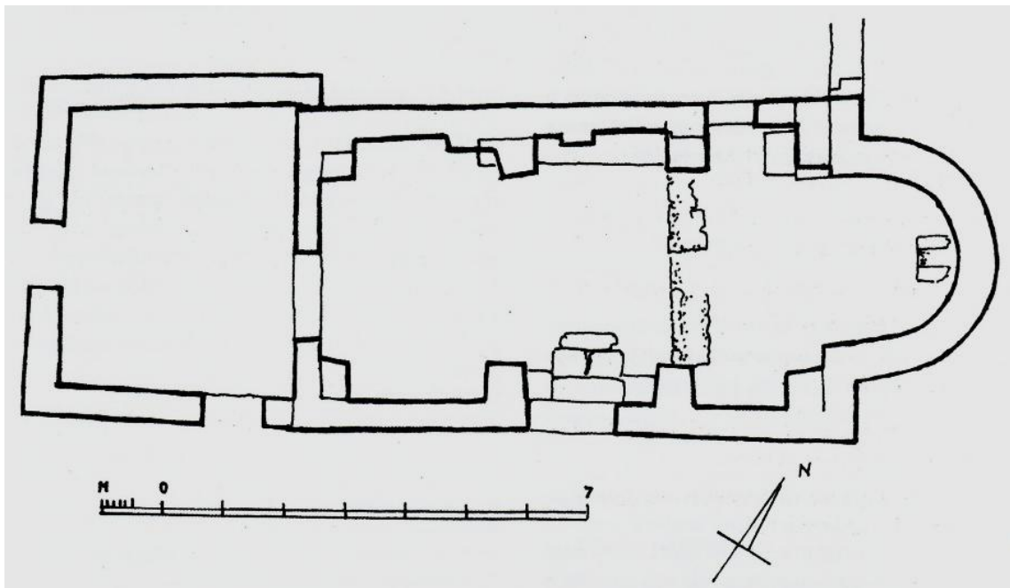
1. Tlocrt ostataka crkve Sv. Ivana u Stivanjem polju kod Sali (I. Petricioli, 1987.)
