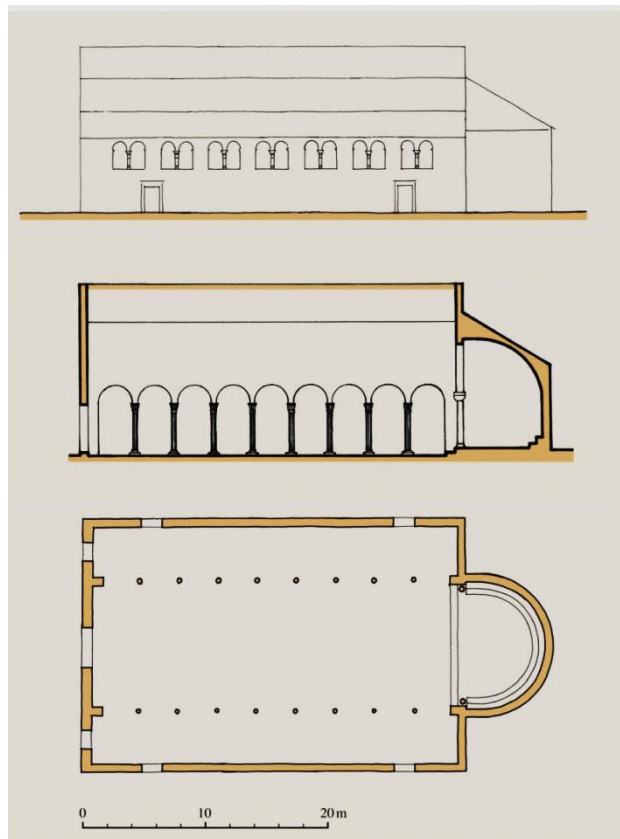
1. Zadar, Sv. Stjepan – tlocrt i grafička rekonstrukcija izgleda ranokršćanske bazilike (P. Vežić, 2005.)
