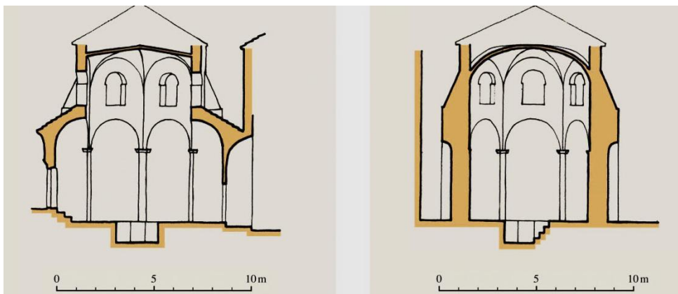
1. Zadar, Sv. Petar – grafička rekonstrukcija poprečnog i uzdužnog presjeka krstionice (P. Vežić, 2005.)
