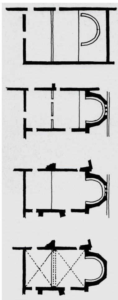
2. Zadar, Sv. Petar – razvojne faze katekumeneja od oratorija do sakristije (P. Vežić, 1990.)
