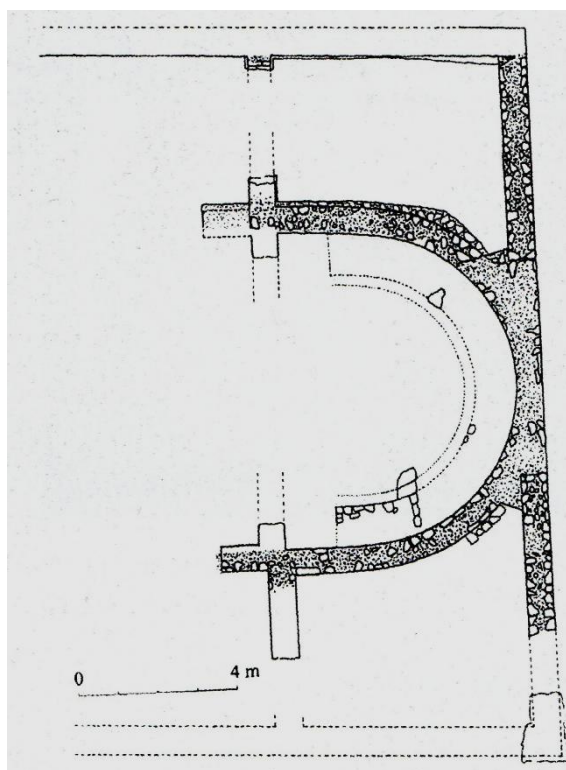
1. Zadar (Relja), Sv. Ivan Krstitelj – tlocrt prezbiterija ranokršćanske bazilike (P. Vežić, 2005.)
