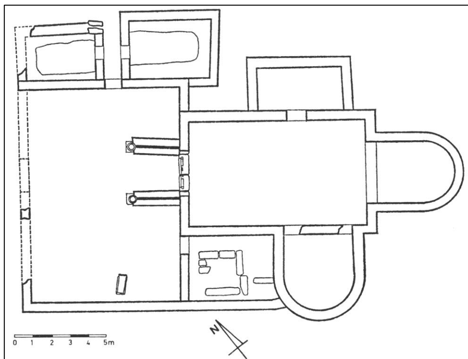
Sl. 11. Muline (Stivan) – tlocrt memorijalnog kompleksa iz 4.-5. st. (prema: M. Suić, 1981.)
