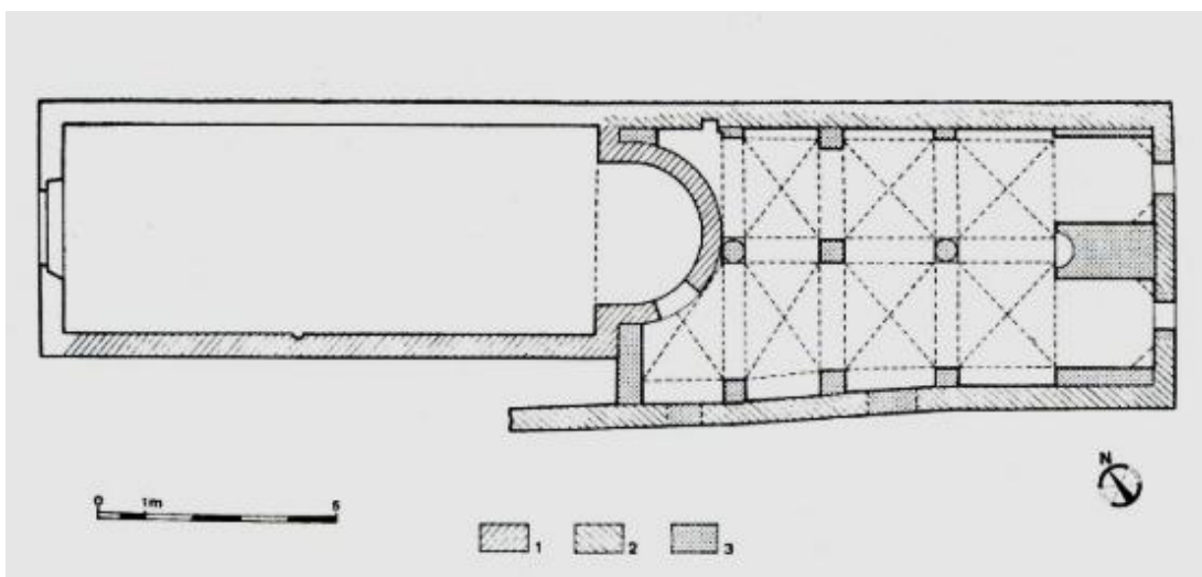
1. Zadar (Iader) – tlocrt povezanih crkava Sv. Andrija i Sv. Petar Stari ( I. Petricioli – S. Vučenović, 1970.)
