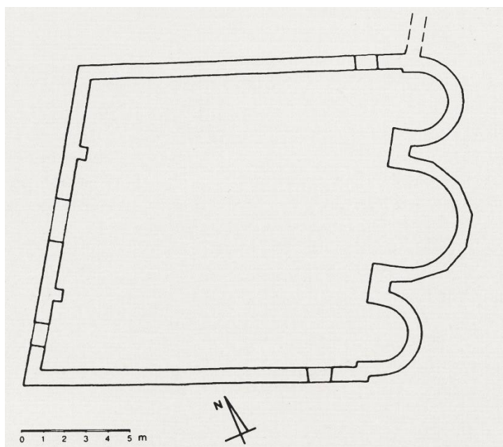
1. Zaton, Sv. Andrija – tlocrt crkve (A. Uglešić, 2002.)
