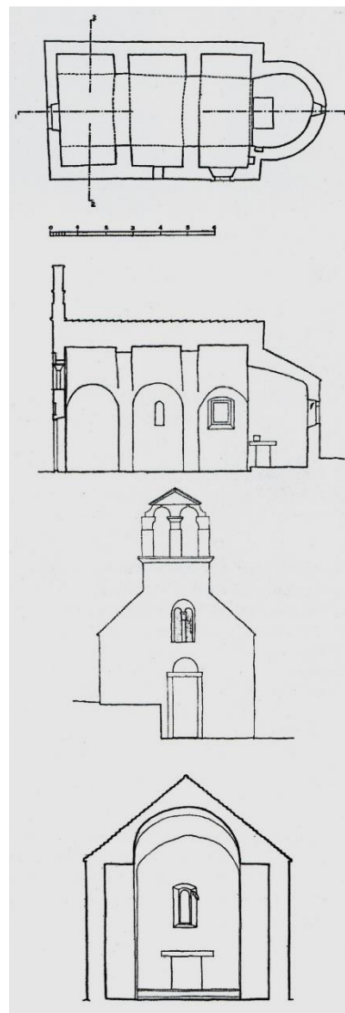
2. Tlocrt, presjeci i pročelje crkve Sv. Andrije u Vrgadi (M. Domijan, 1983.)
