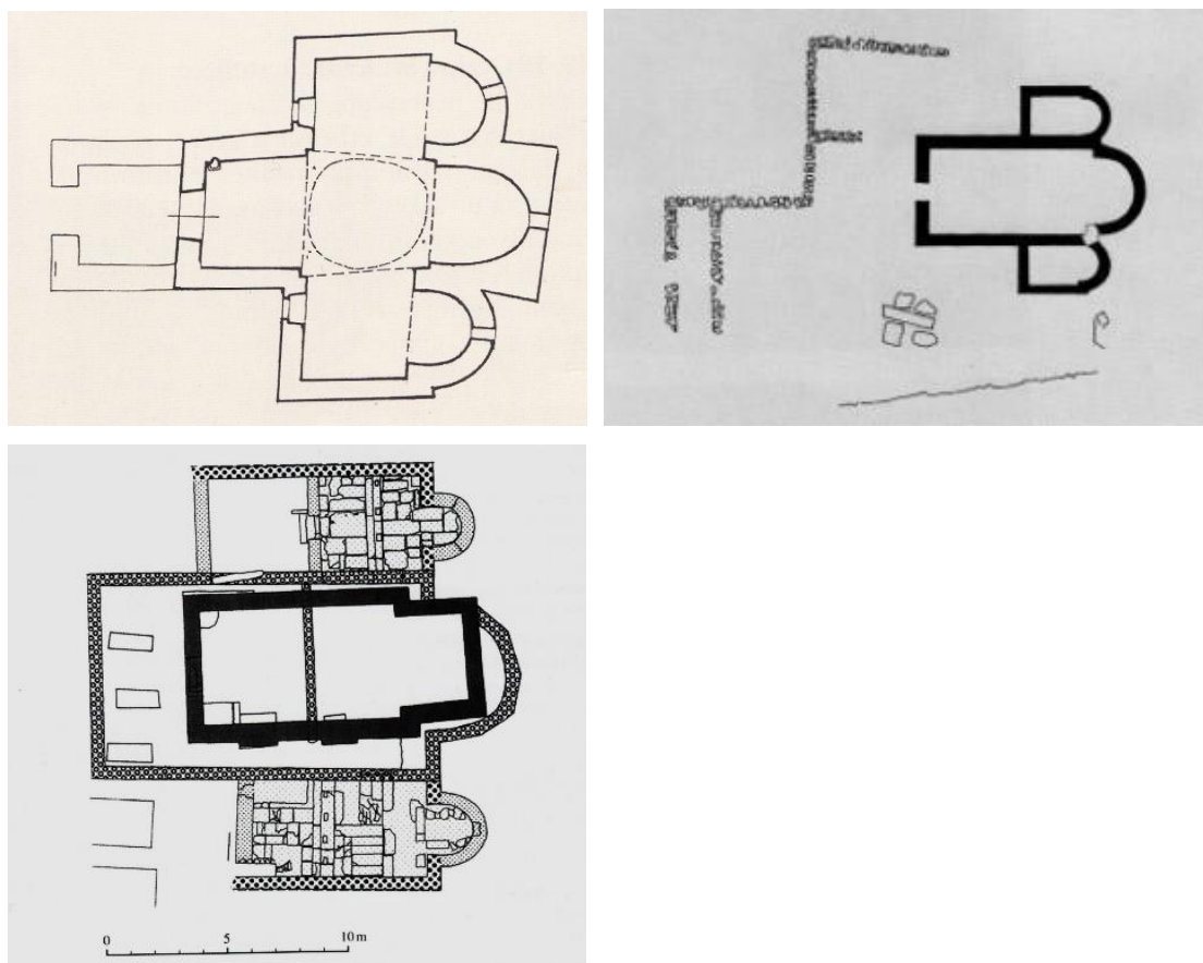
Sl. 24. Troapsidalno svetište kod crkve Sv. Križa u Ninu (prva u gornjem redu) te primjeri troapsidalnog svetišta koje nastaje dodavanjem pomoćnih prostorija u predromanici i romanici: Begovača u Biljanima Donjim, Sv. Martin u Lepurima (u donjem redu), (prema: N. Jakšić, 1989., 2000.)
