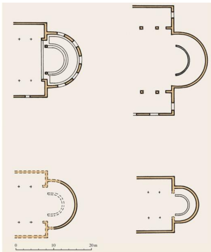
Sl. 9. Apside sa subselijem i prolazom iza njih: Zadar – Katedrala, Salona – Katedrala, Novalja – Sv. Marija, Rab – Sv. Ivan Evanđelist (prema: P. Vežić, 2005.)
