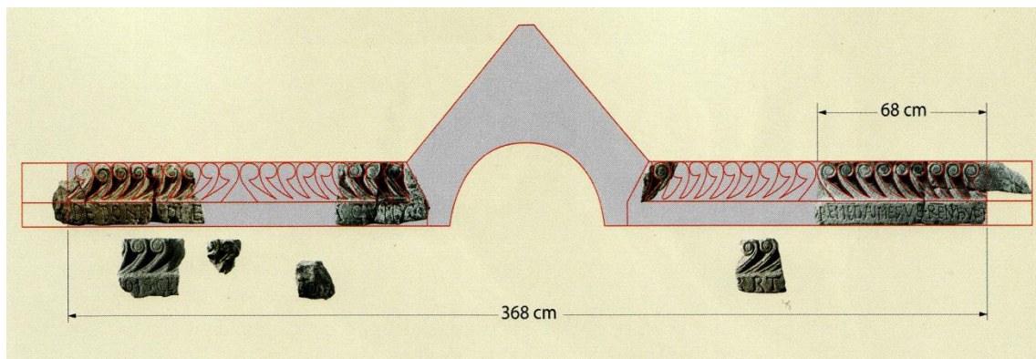
Sl. 40. Biljane Donje, Begovača – rekonstrukcija luka predromaničke ograde svetišta s jednim središnjim zabatom (prema: I. Josipović, 2012.)
