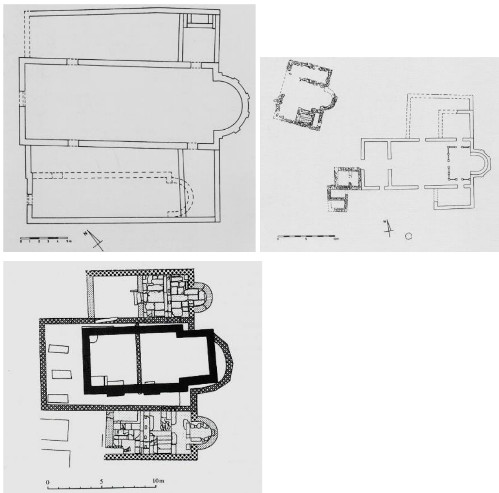
Sl. 13. Tlocrti kompleksnih/složenih(naronitanskih) crkava u zadarskoj okolini, od lijeva na desno: Sv. Asel u Ninu, Sv. Bartolomej (Crkvina) u Galovcu, Sv. Martin u Lepurima (prema: A. Uglešić, 2002., J. Belošević, 1997., N. Jakšić, 2000.)
