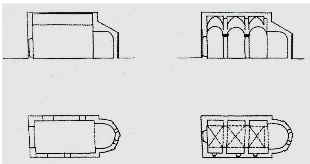
2. Ošljak, Sv. Marija (Vela Gospa) – usporedni tlocrt i presjek ranokršćanske i predromaničke faze crkve (P. Vežić, 1992.)
