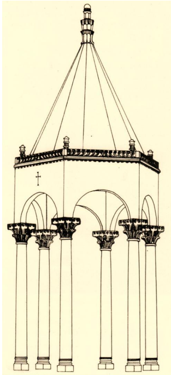
Sl. 48. Galovac, Crkvina (Sv. Bartolomej) – pretpostavljeni izgled predromaničkog ciborija šestorostrane tlocrtne osnove (prema: J. Belošević, 1993.)
