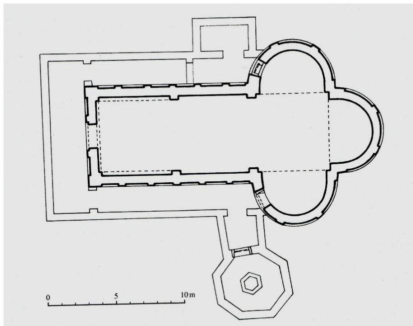
1. Pridraga, Sv. Martin – tlocrt crkve (P. Vežić, 2005.)
