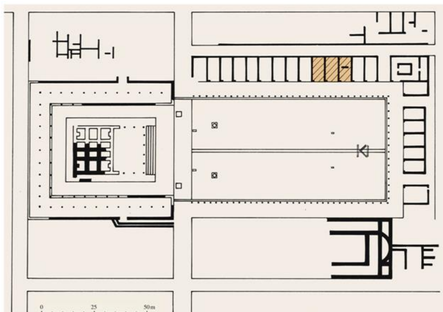
Sl. 4. Grafička rekonstrukcija rimskog kapitolija i foruma te kršćanskog oratorija (označeno) u sklopu taberna (prema: P. Vežić, 2005.)
