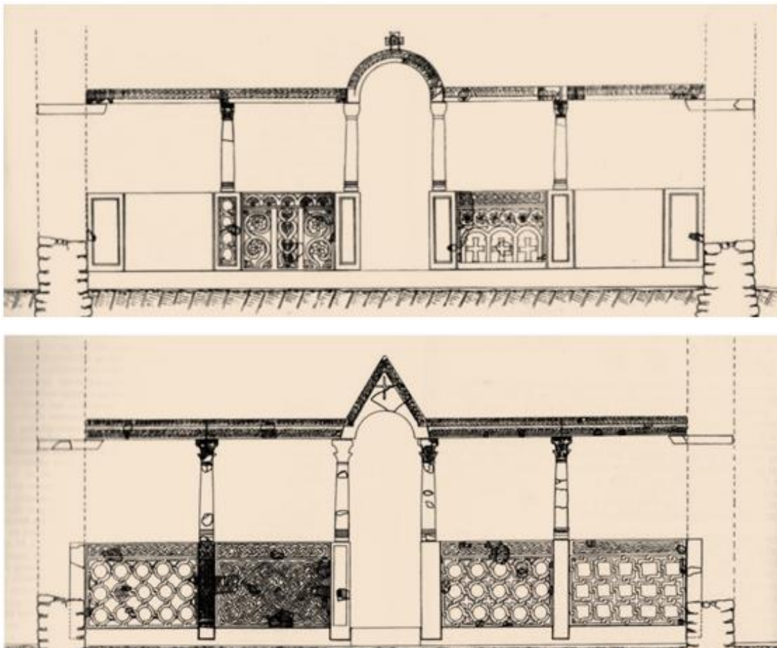
Sl. 41. Galovac, Crkvina – grafička rekonstrukcija pretpostavljenog izvornog izgleda ograde svetišta iz prve predromaničke obnove (gore), i druge predromaničke obnove (dolje) (prema: J. Belošević, 1997.)
