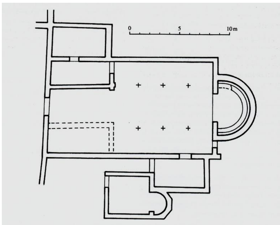
2. Muline (o. Ugljan), Sv. Ivan Krstitelj – tlocrt ranokršćanske bazilike s aneksima (M. Suić, 1960.)
