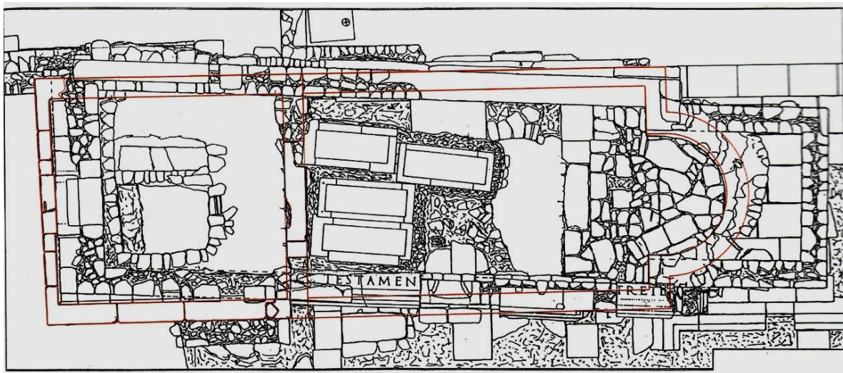
1. Podgrađe ( Asseria ), Sv. Duh – tlocrt istraženih ostataka unutar i uokolo crkve s pretpostavljenim položajem ranokršćanske crkve (označeno crvenom bojom) (A. Uglešić, 2002.)
