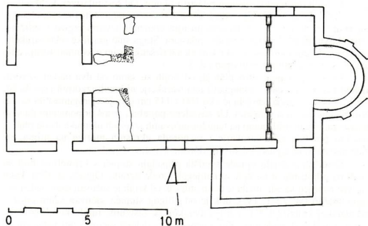
1. Galovac, Crkvina – tlocrt reducirane ranokršćanske crkve u vrijeme prve predromaničke faze (J. Belošević, 1997.)
