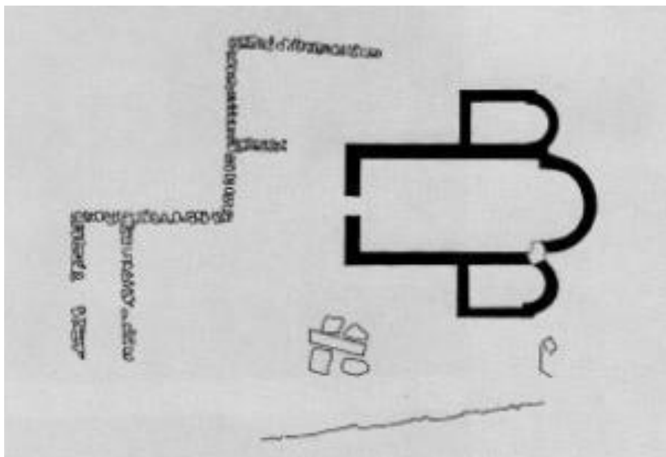
2. Biljane Donje, Begovača (Crkvina) – tlocrt srednjovjekovne crkve (N. Jakšić, 1989.)
