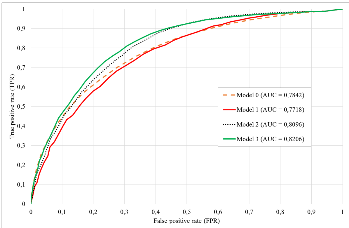
Slika 37. ROC krivulje izrađenih modela pogodnosti terena jaruženju napravljene na temelju 120 jaruga kartiranih OBIA pristupom
