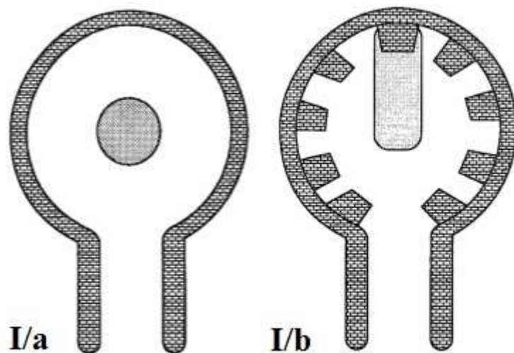
Sl. 18. Tlocrt peći tipa I/a s centralno postavljenim stupom i tipa I/b s radijalno postavljenim pilastrima, preuzeto iz: Šimić–Kanaet 1996: 158–159
