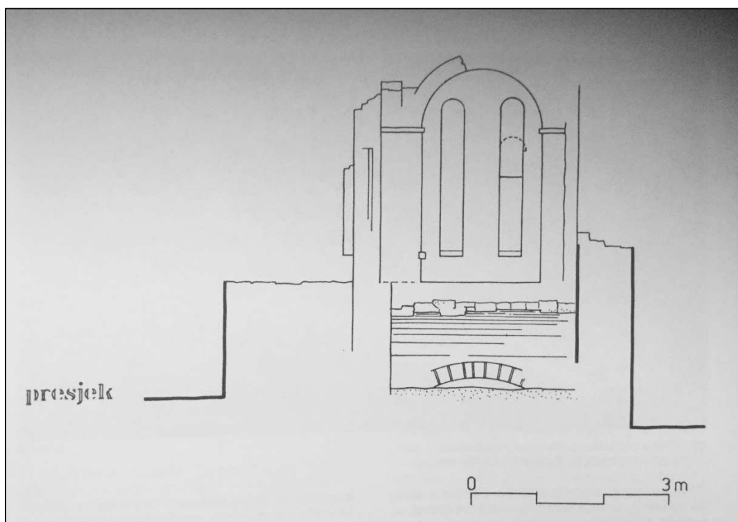
Slika 47: Presjek predromaničke crkve sv. Mihovila na Mrkanu (prema: I. FISKOVIĆ, 1980, 248.)
