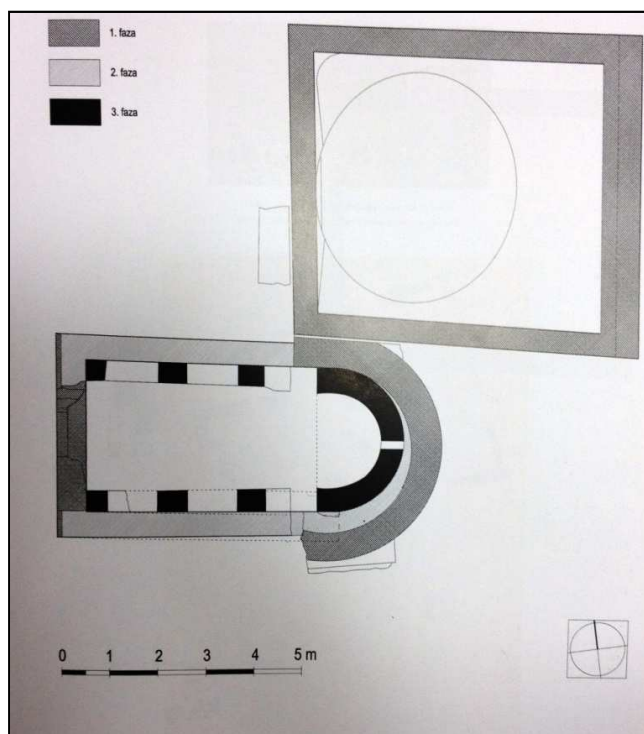
Slika 2: Tlocrt crkve i cisterne s fazama izgradnje (prema: D. RADIĆ, Z. TOLJA, 2010, 173.)
