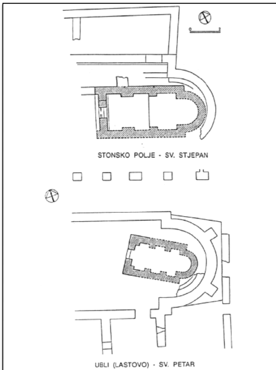
Slika 13: Usporedba tlocrtne situacije sv. Stjepana u Barama i sv. Petra u Ublima (prema: R. MENALO, 2009, 275.)
