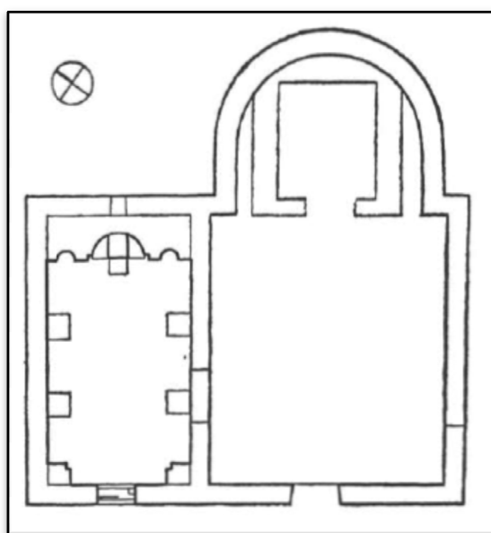
Slika 17: Tlocrt starokršćanske crkve sv. Petra na Zamlinju (prema: I. FISKOVIĆ, 1985, 146.)
