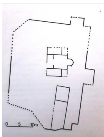
Slika 31: Tlocrt kasnoantičke utvrde sa starokršćanskom crkvom (prema: J. JELIČIĆ RADONIĆ, 1997, 150.)
