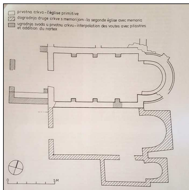
Slika 37: Crkva Polače - Mljet (prema: I. FISKOVIĆ, 1988, 201.)
