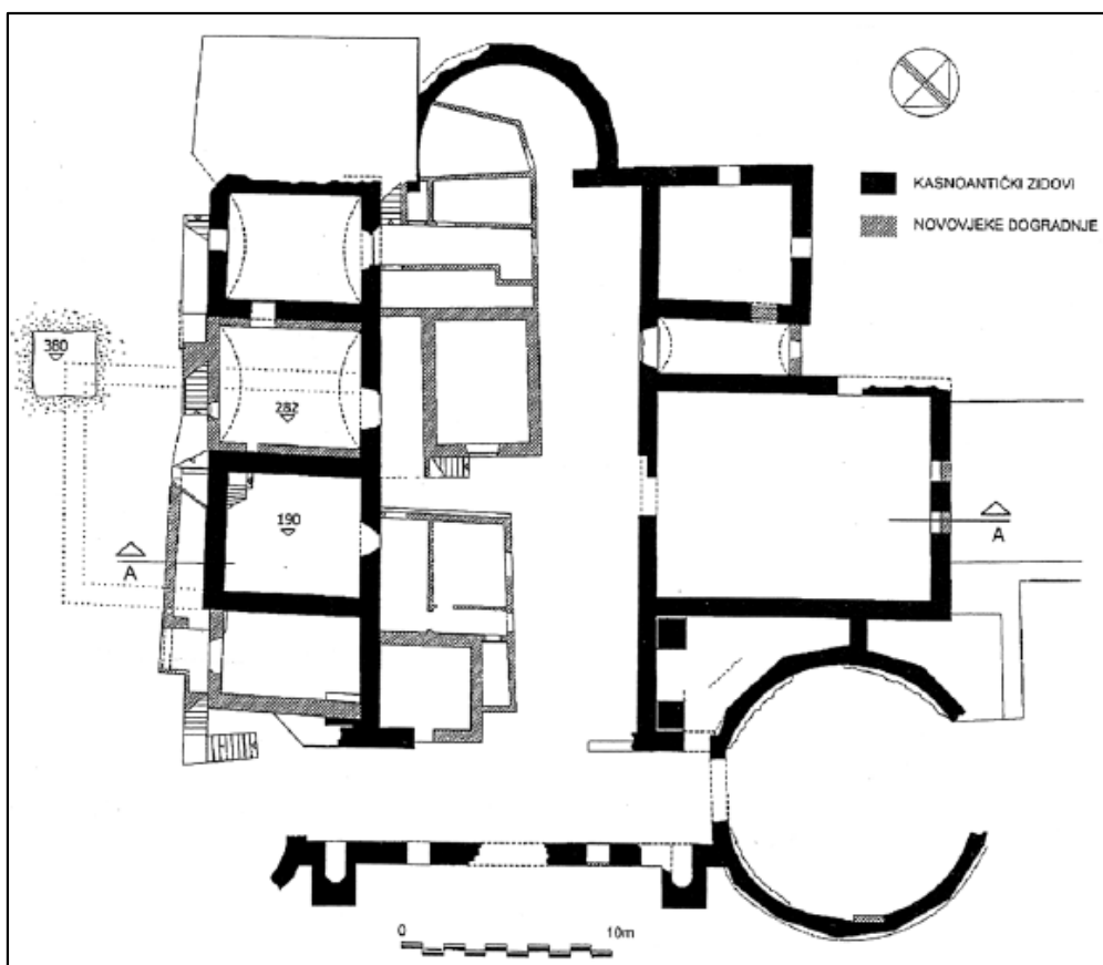
Slika 35: Tlocrt palače prema I. Fiskoviću i J. Stošiću (preuzeto iz: T. TURKOVIĆ, 2011, 202.)
