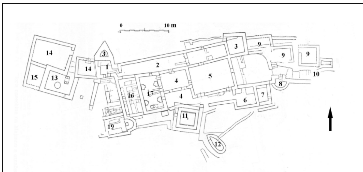
Slika 23: Tlocrt kompleksa na Majsanu (prema: C. FISKOVIĆ, 1984, 23.) 1: glavni ulaz, 2: hodnik, 3: obrambene kule, 4: zajedničke prostorije, 5: središnji atrij, 6: kuhinja, 7: kupaonica, 8: latrina, 9: spavaće sobe, 10: istočni ulaz, 11: cisterna, 12: bunar, 13: turnjačica, 14: skladište, 15: trijem uz ulaz i luku, 16: kasnoantičko groblje, 17: starokršćanska memorija, 19: ranosrednjovjekovna crkvice
