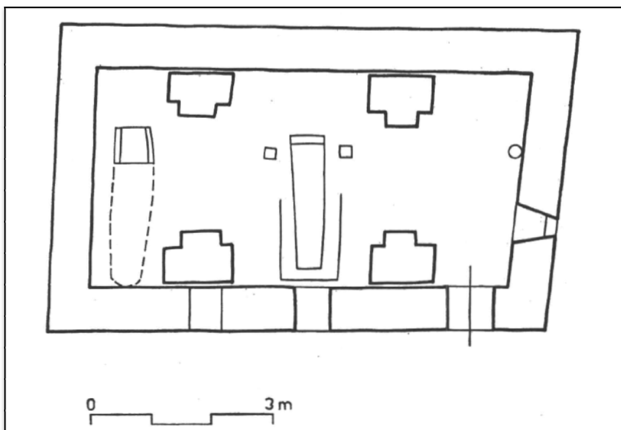
Slika 20: Tlocrt starokršćanske memorije na Majsanu (prema: C. FISKOVIĆ, 1983, 73.)
