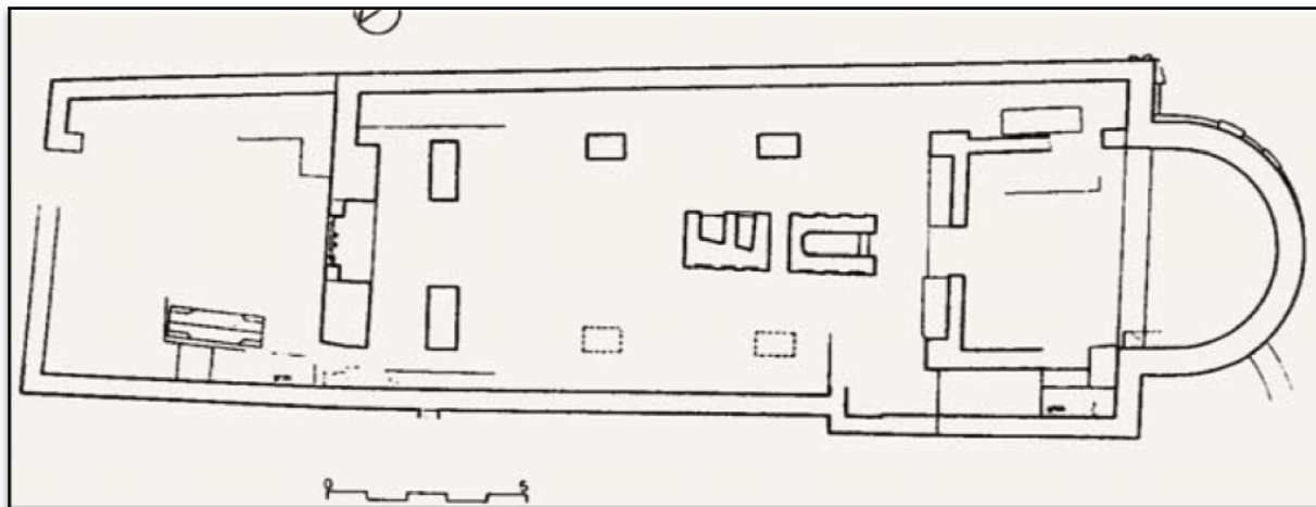
Slika 15: Tlocrt crkve sv. Mandaljene na Gorici (prema: Hrvati i Karolinzi II , 337.)
