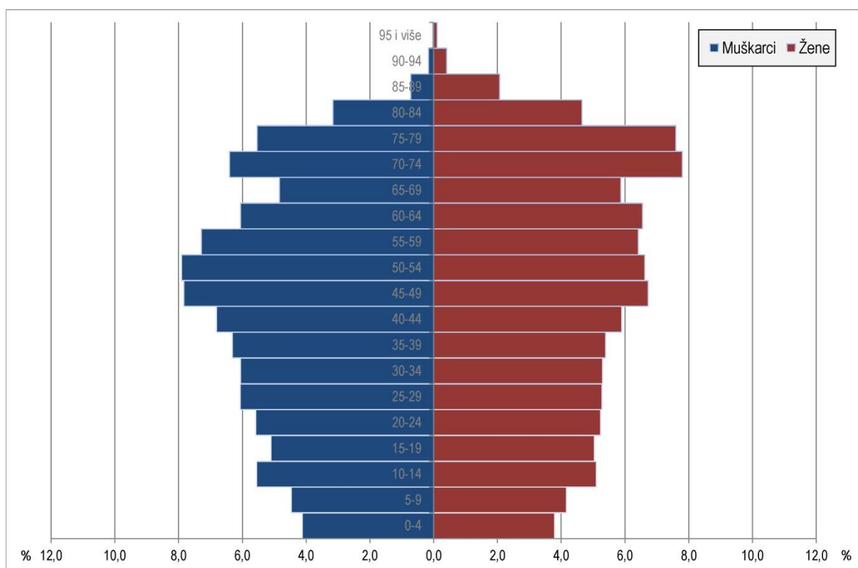
Slika 66. Dobno-polna piramida stanovništva Ličko-senjske županije 2011. godine (izvor: Popis stanovništva, kućanstava i stanova 2011. godine, Stanovništvo prema spolu i starosti po naseljima , DZS, Zagreb.)
