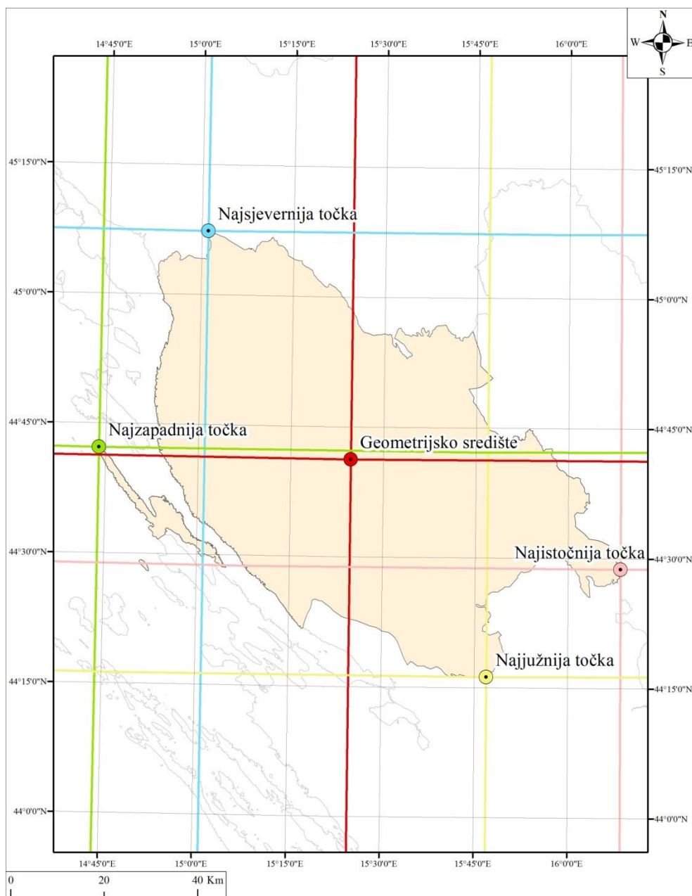
Slika 2. Geografski smještaj Ličko-senjske županije
