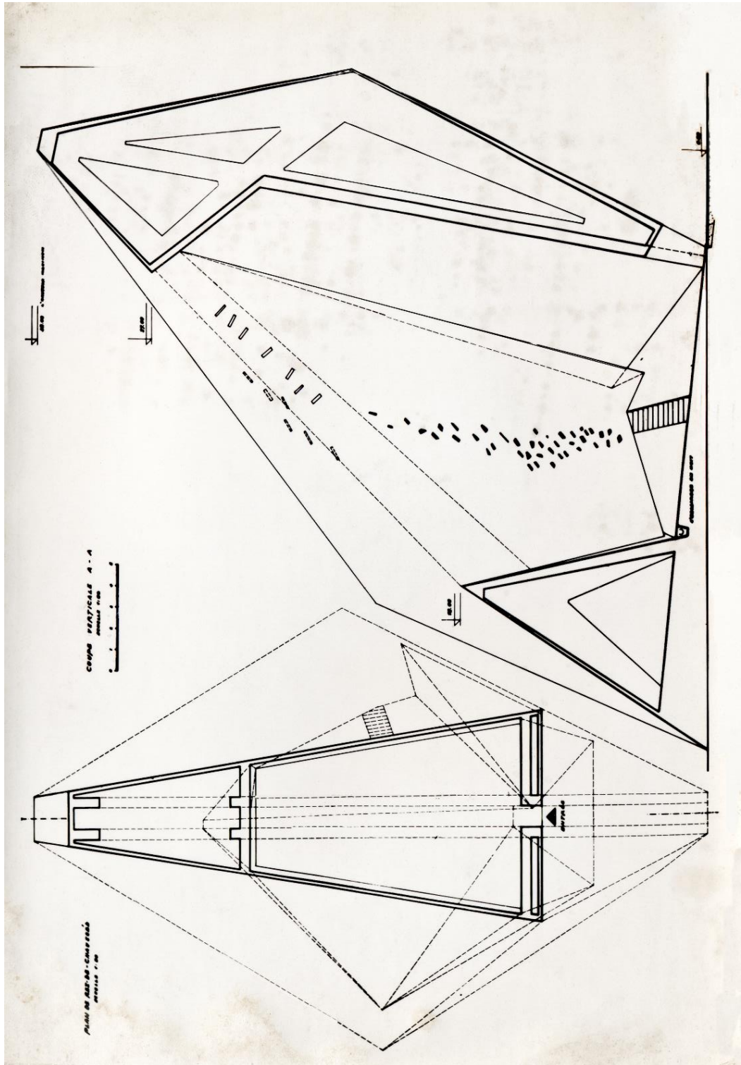
Slika 4. Prvi natječajni projekt za spomenik žrtvama fašizma u bivšem koncentracijskom logoru Dachau, Dušan Džamonja i Ninoslav Kućan, 1958.–1959., presjek. Izvor: Arhiva Dušana Džamonje.
