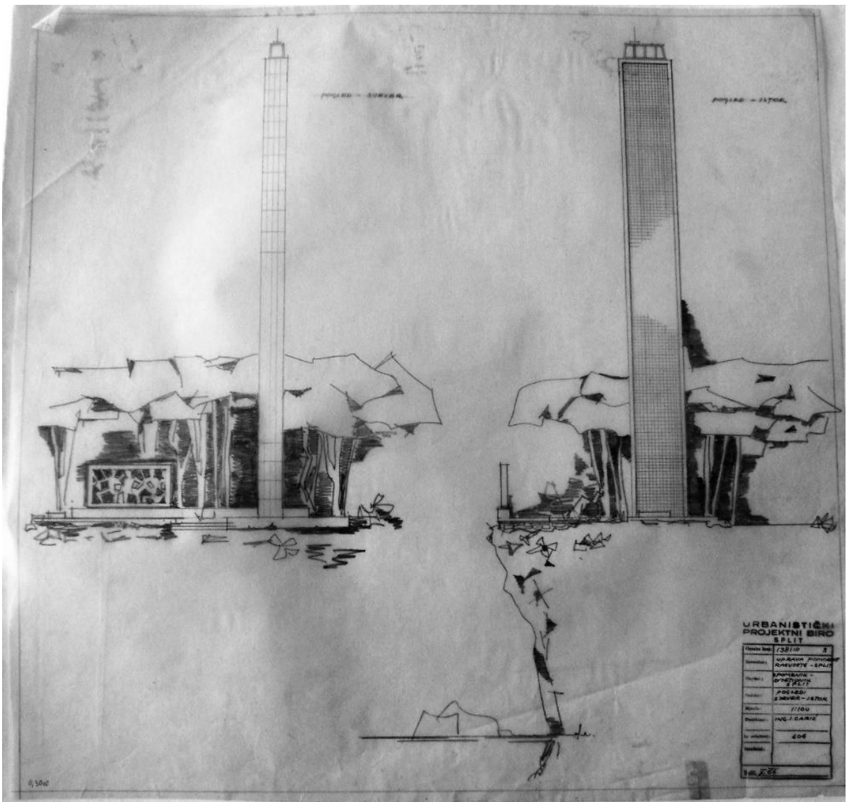
Slika 140. Spomenik palim pomorcu , Split, Andrija Krstulović, Ivan Carić, Budimir Pervan, Branko Franičević, 1958. Izvor: DAST.
