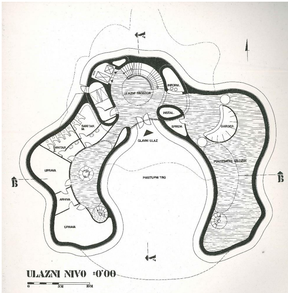
Slika 32. Spomenik ustanku naroda Korduna i Banije, Petrova gora, Vojin Bakić i Berislav Šerbetić, 1981., tlocrt ulaznog nivoa. Izvor: Projekt spomenika... (1981.), 41.
