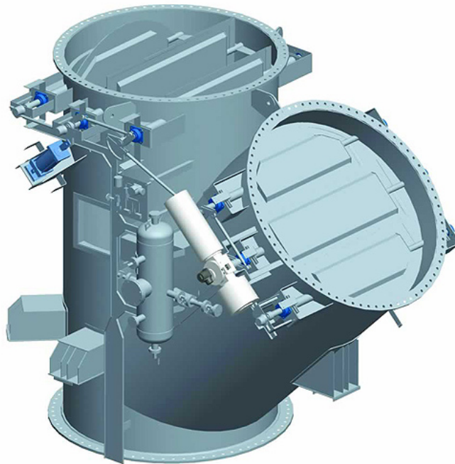
Slika 7. Klapne generatora pare na ispušne plinove [11]
