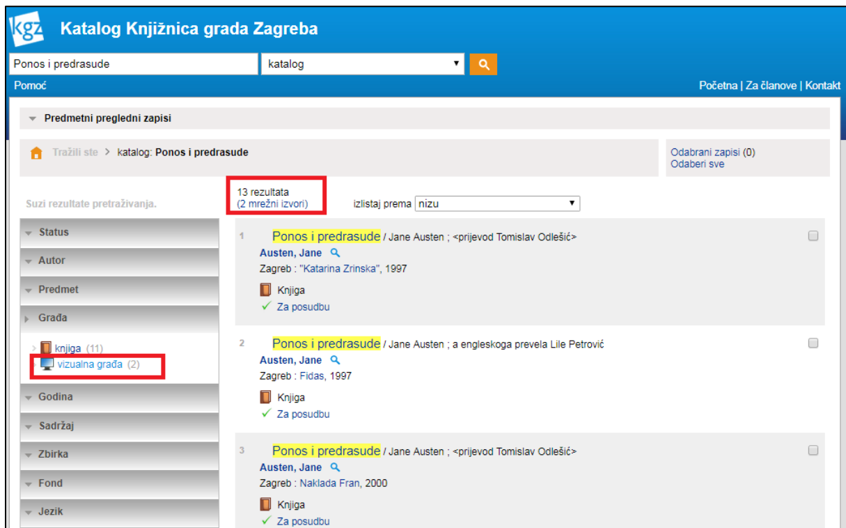
Slika 10. Pronalaženje entiteta
