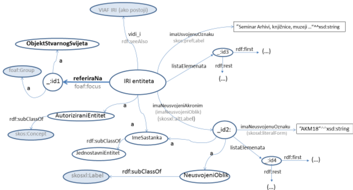
Slika 16. Shema modeliranja odnosa između konceptualnog entiteta (instance klase oap:ImeSastanka ) i objekta stvarnog svijeta (instance klase oap:ObjektStvarnogSvijeta ) na kojem konceptualni entitet referira.
