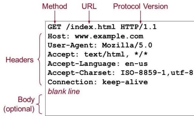
Slika 19 Objašnjenje HTTP zahtjeva[30]
