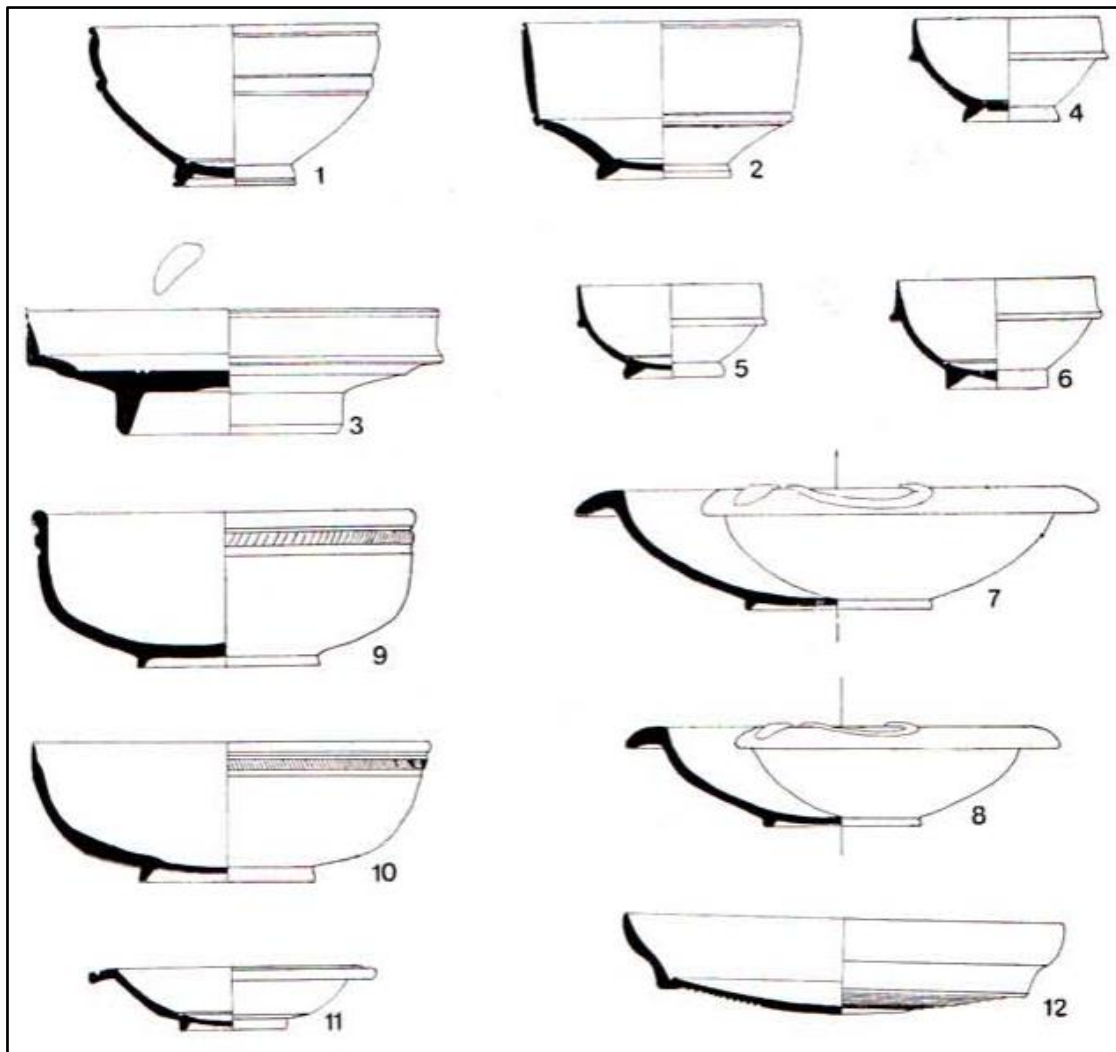
Slika 15. Prikaz nalaza terre sigillate (prema: Makjanić, R., 1985, TAB V.)
