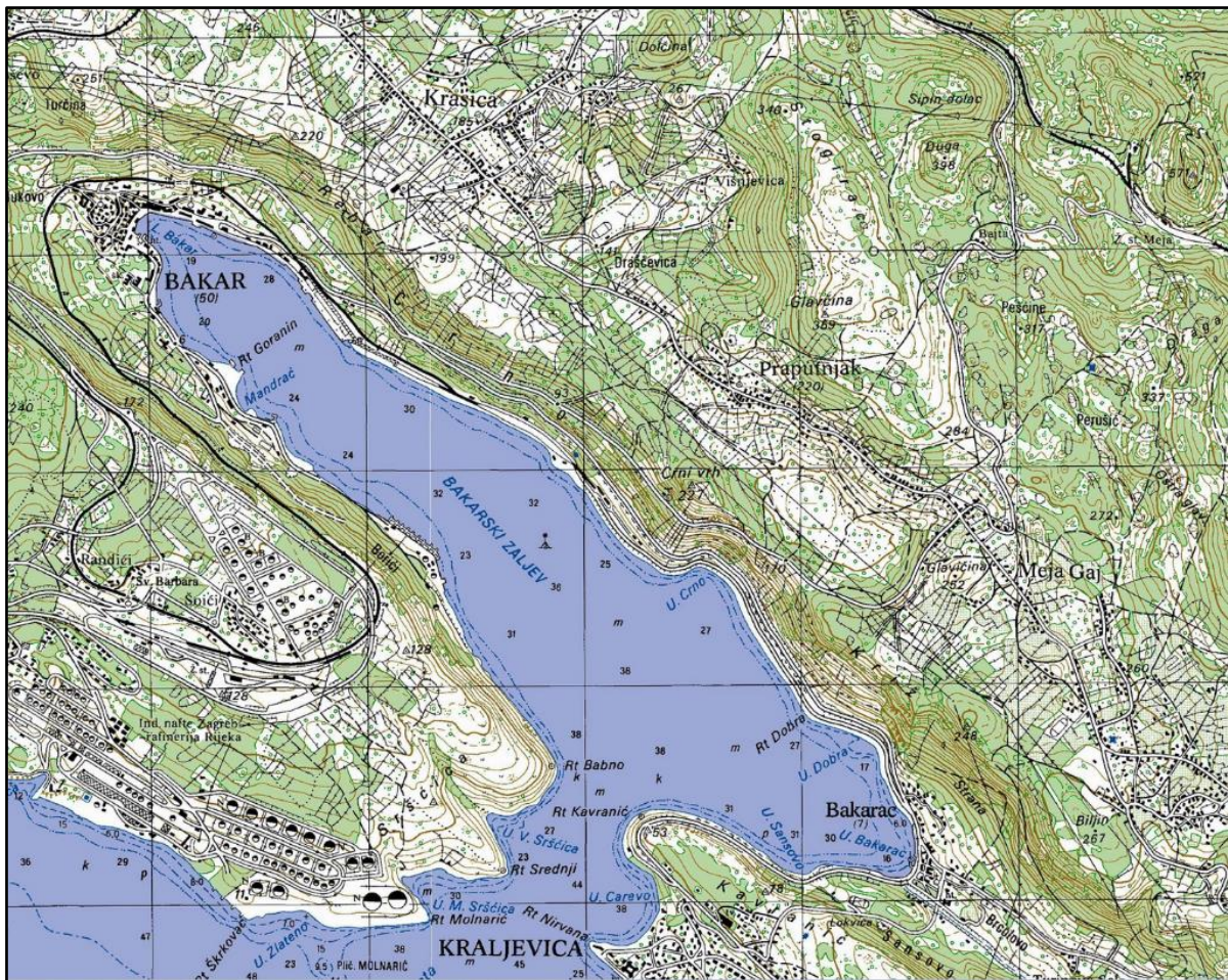
Slika 1. Topografska karta Bakarskog zaljeva i okolice
