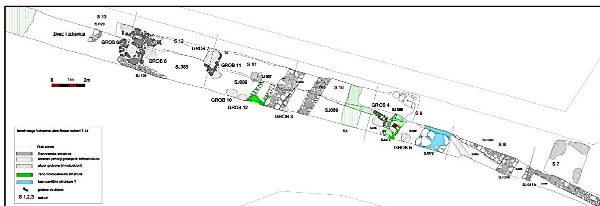
Slika 18. Skica rimskih zidanih, kasnoantičkih, novovjekovnih konstrukcija i rimskih ukopa (prema: Makarun, M., 2023, 11.)
