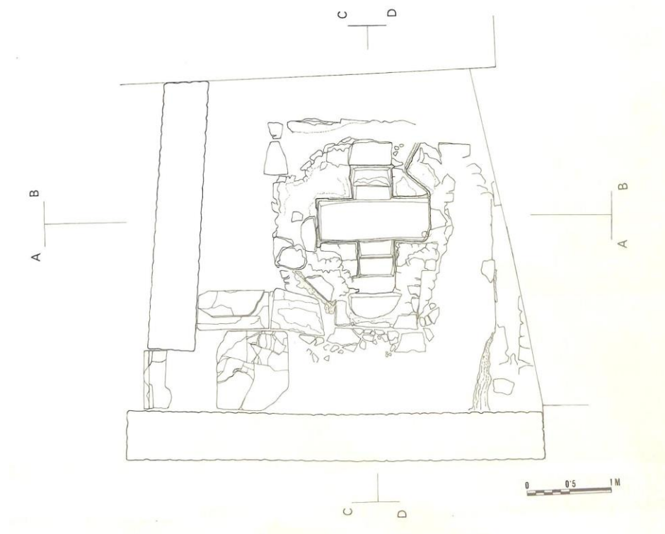
Slika 14. Tlocrt krsnog zdenca (J. Jeličić-Radonić, 1994, 23.)
