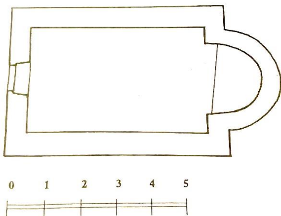
Slika 40. Tlocrt crkve sv. Marije Magdalene
