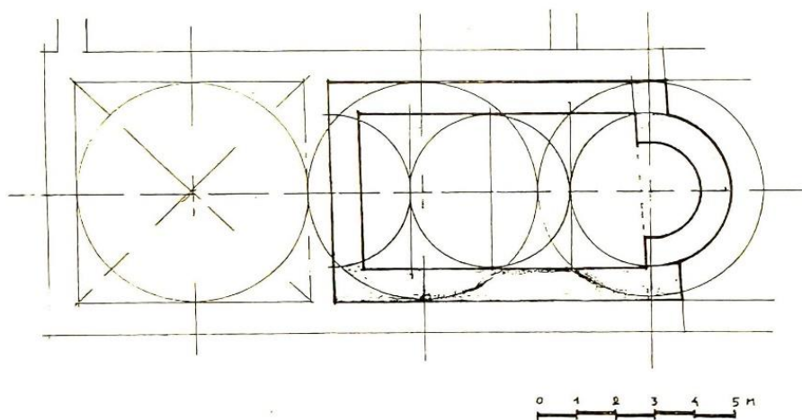
Slika 28. Tlocrt, proporcijski odnosi i rekonstrukcija gradnji u kapeli sv. Prospera u Hvaru
