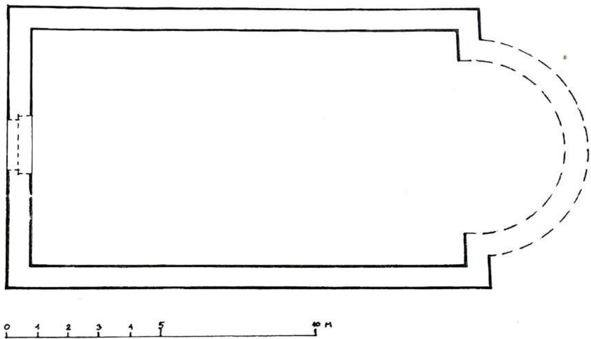
Slika 41. Tlocrt crkve sv. Ciprijana, Vrisnik
