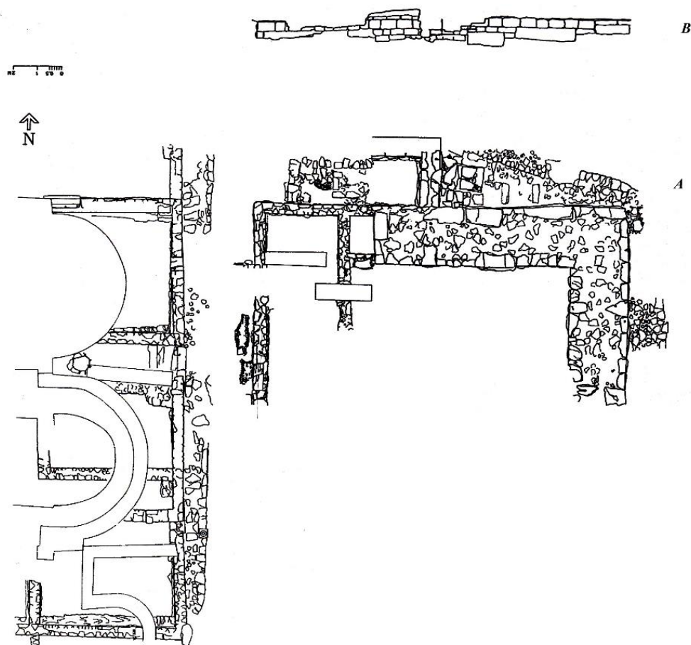
Slika 3. Tlocrt istočnih gradskih bedema i sklopa grčke arhitekture pored crkve sv. Ivana (J. Jeličić-Radonić, 1995, 58.)
