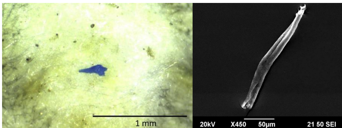
Slika 7. a) mikroplastični fragment iz tijela dagnje (Norveška) (izvor: Bråte i sur., 2018.); b) jedno od mikrovlakana iz tijela dubokomorskih (>2200 m) bentičkih beskralježnjaka (izvor: Courtene-Jones i sur., 2017.).
