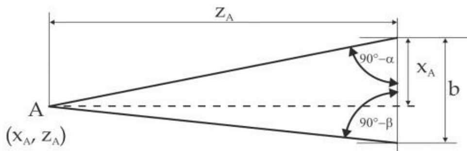
Slika 9. Mjerenje udaljenosti triangulacijom (preuzeto od Guidi i Remondino, 2012)
