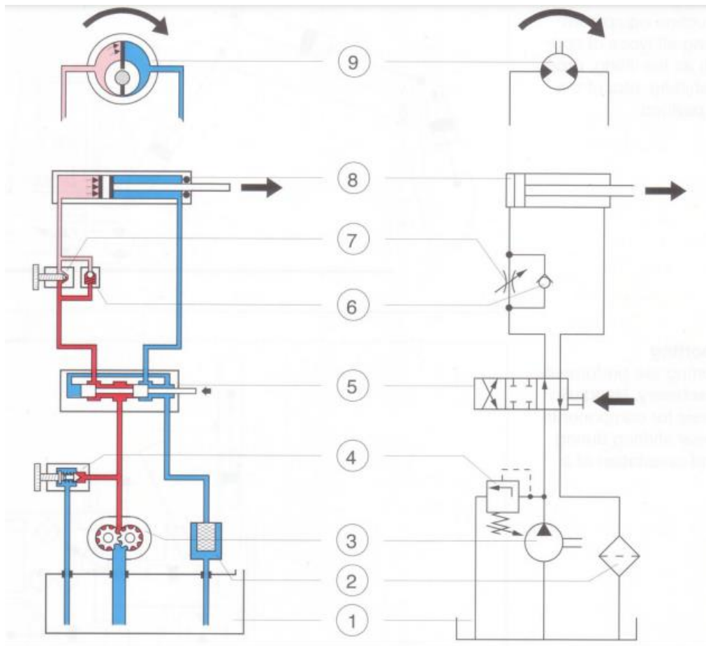
Slika 4. Dijelovi hidrauličkog sistema vitla [6]
