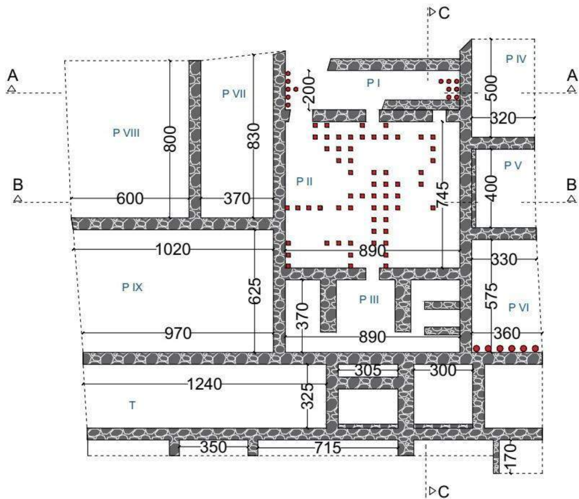
Slika 8. Tlocrt iskopane arhitekture sa označenim prostorijama 1977. god. (Izradio M. Rašić prema originalu odgovernog arhitekta Ferhada Mulabegovića 1978. god.)
