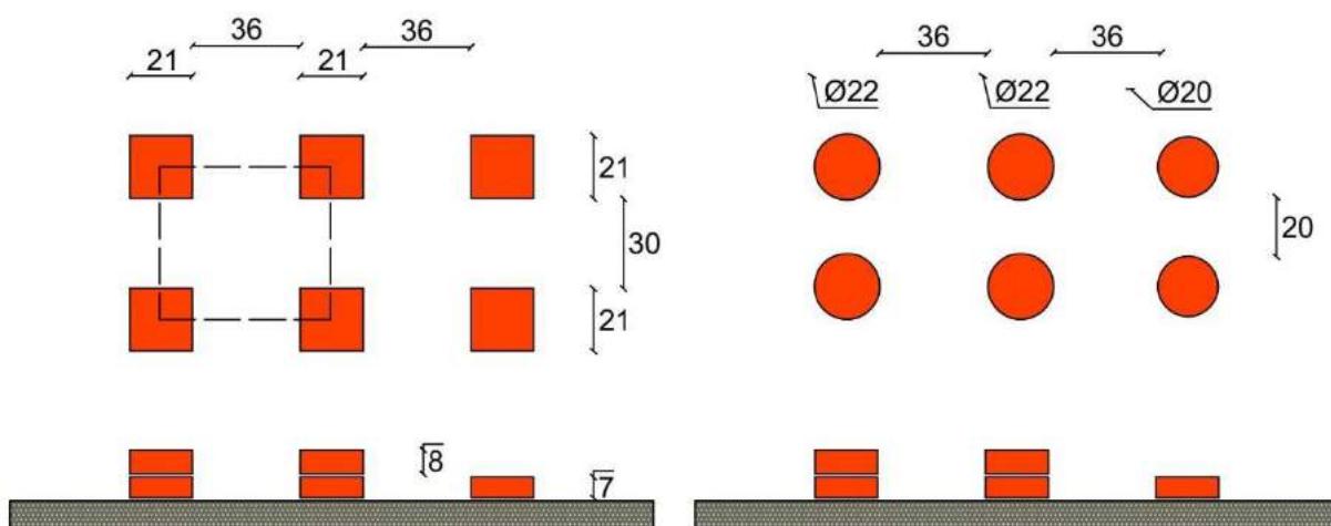
Slika 9. Pozicija i presjek suspenzura hipokausta iz Prostorije I i II. (Izradio M. Rašić prema originalu odgovornog arhitekta Ferhada Mulabegovića 1978. god.)
