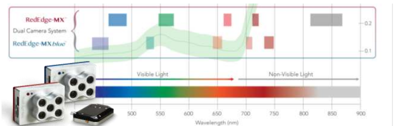
Slika 6. MicaSense RedEdge-MX Dual Camera i valne duljine spektralnih kanala (URL6)
