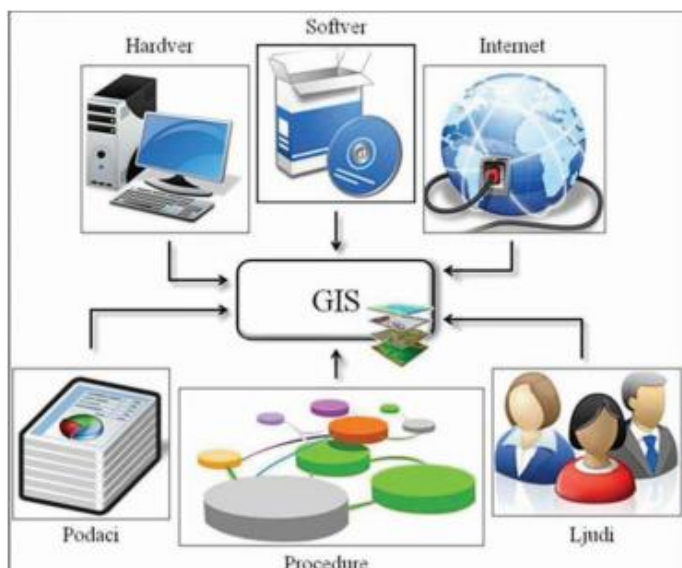
Slika 4. Komponente GIS-a
