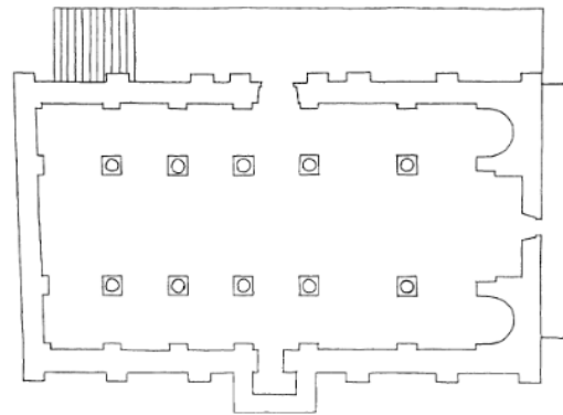
Slika 54: Tlocrt crkve Sv. Nediljice (P. VEŽIĆ, 1999, 11)
