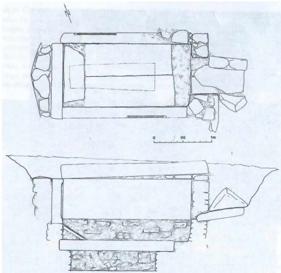
Slika 8 – tlocrt kasnoantičke grobnice u Dugopolju (izvor: N. CAMBI, 1994., 152., slika 4.)
