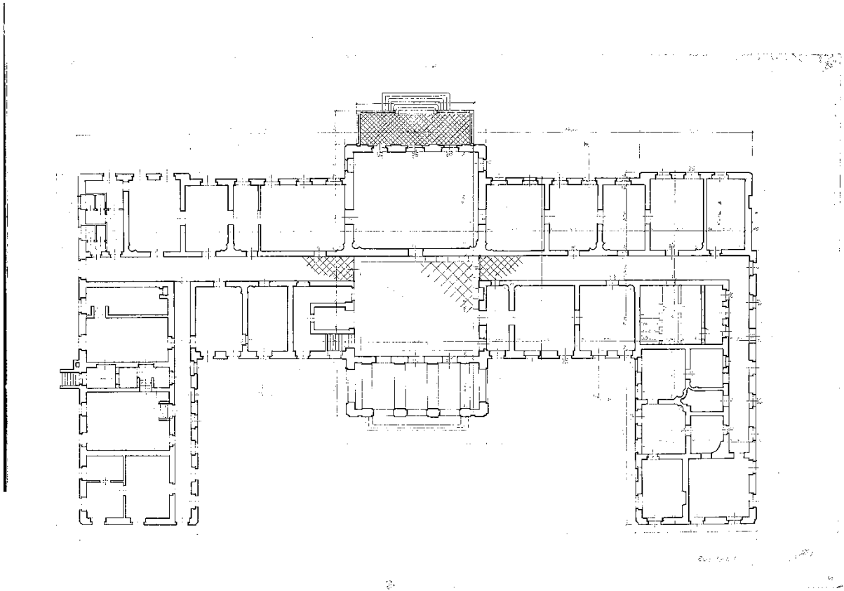
Prilog 3. Tlocrt dvorca Pejačević u Retfali, izvor: MK-UZKB-MF-1269
