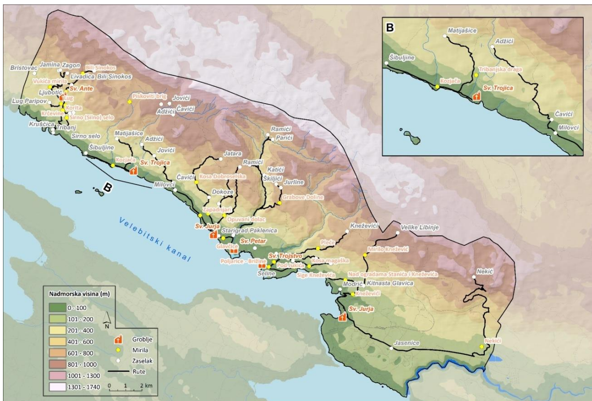
Slika 37. Prikaz prostornog obuhvata promatranog područja s pripadajućim mirilima i putovima (s naglaskom na mirila naselja Tribanj Šibuljina: Kozjača i Tribanjska draga) Izvor: izrađeno na temelju: središnji registar prostornih jedinica (SRPJ), EU-DEM, Geofabrik, terensko istraživanje (GPS)
