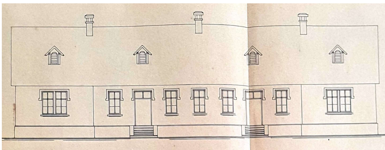
Prilog 4.4. Tocrt i pročelje Oružničke i Kotarske ispostave u Kupresu (ABH, ZVS)
