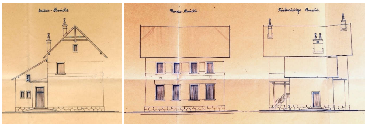
Prilog 7.31. Plan za 1909. Narodne osnovne škole u Zloselu – Suhopolje, nastao u listopadu 1908. (ABH, Građevinski odjel) 858
