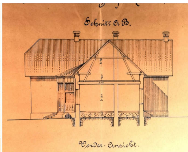
Prilog 7. 28. Projekt Narodne osnovne škole u Kupresu (ABH)
