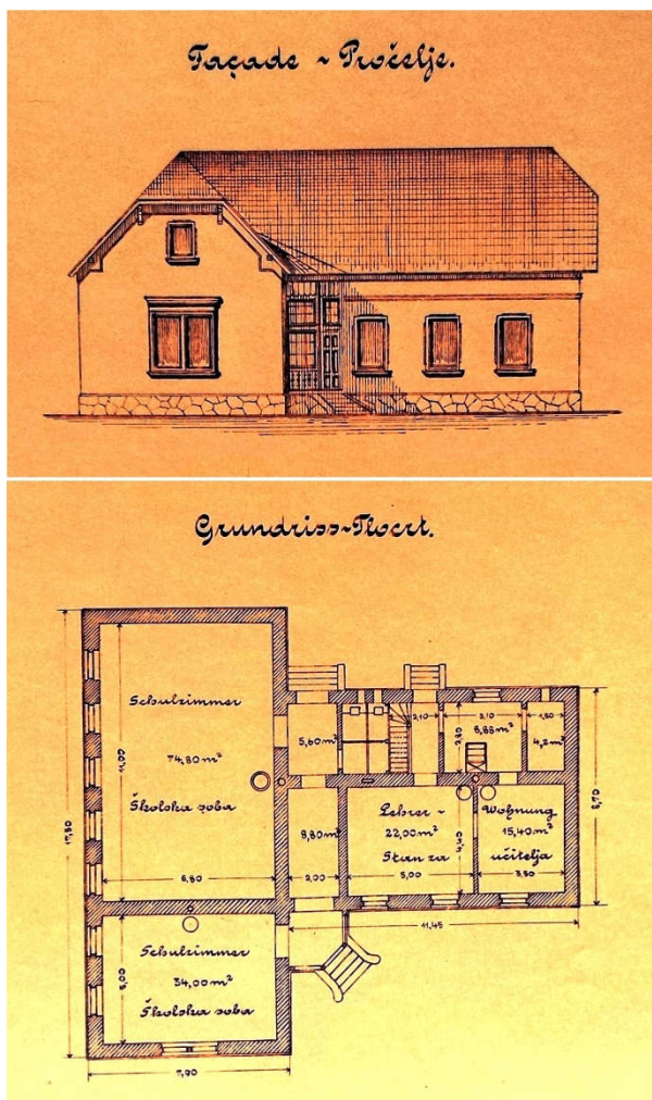
Prilog 7. 28. Projekt Narodne osnovne škole u Kupresu (ABH)
