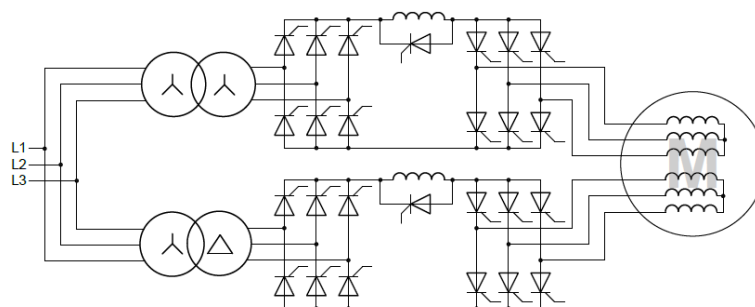
Slika 8. Sinkrokonverter u para-12-pulsnoj konfiguraciji
