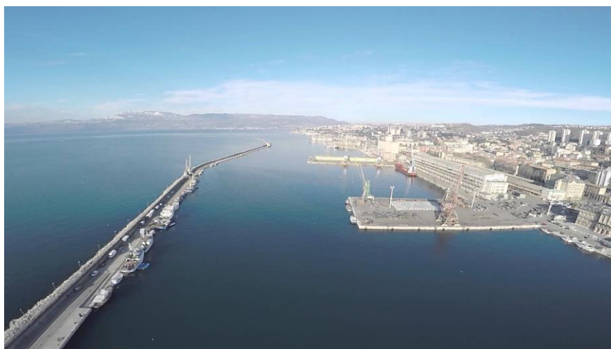
Imagen 10. Rompeolas “Mololongo”
