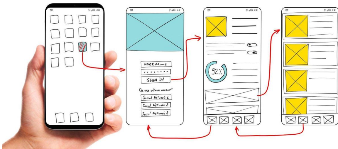
Slika 6 Primjer wireframing-a [11]
