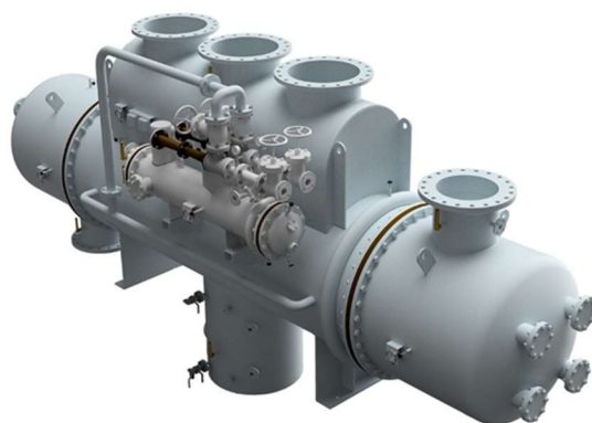
Slika 25. Parni kondenzator [21]
