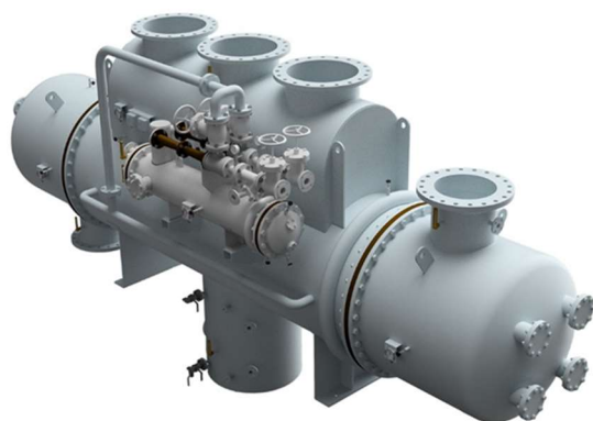
Slika 25. Parni kondenzator [21]
