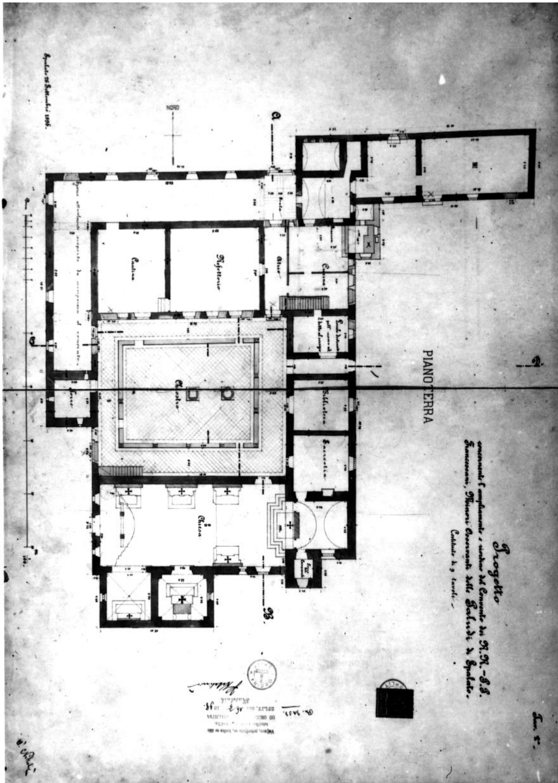
Slika 14. Tlocrt poljudskog samostana (1896.)
