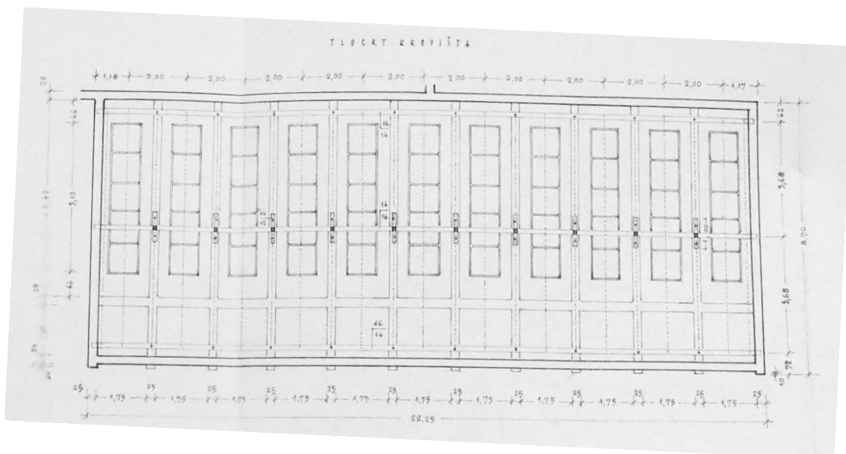
Slika 18 Tlocrt krovništva (dio sveukupnog nacrt projekta) (Izvor: Arhiva SGIMV)
