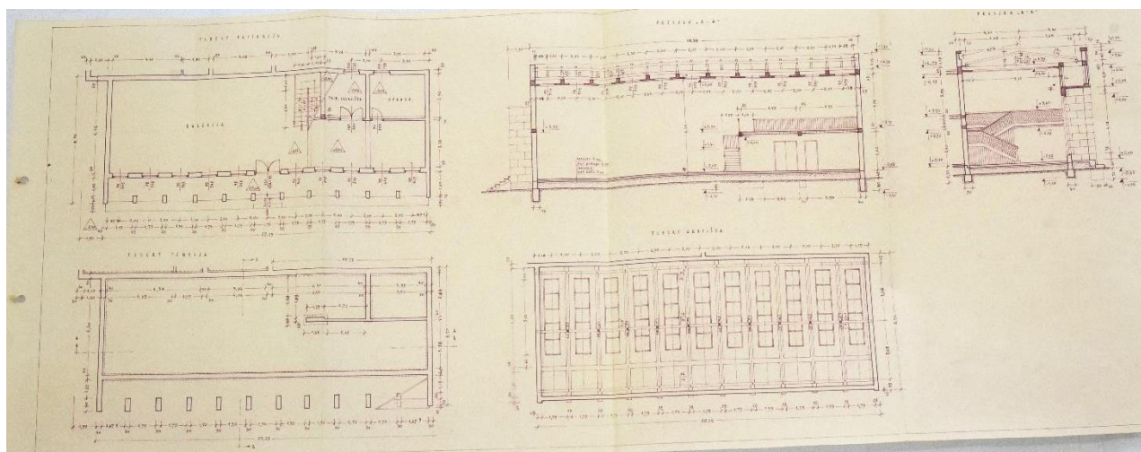
Slika 12 Tlocrti Rudolfa Varge za zgradu Galerije iz 1969. godine (Izvor: Arhiva SGIMV)
