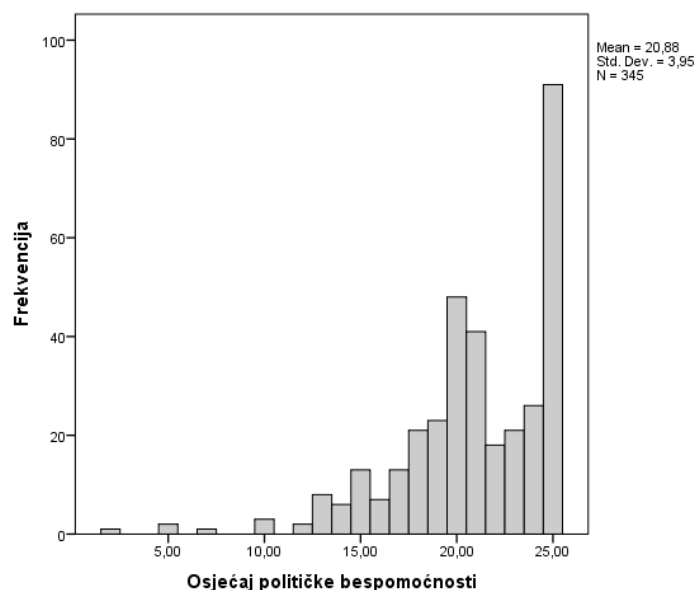
Prikaz 9.4: Distribucija frekvencija za varijablu osjećaja političke bespomoćnosti prije provedene transformacije
