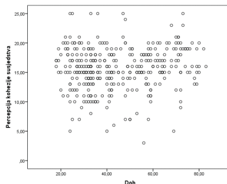
Prikaz 16.3. Dijagram raspršenja za varijable dobi i percepcije susjedske kohezije
