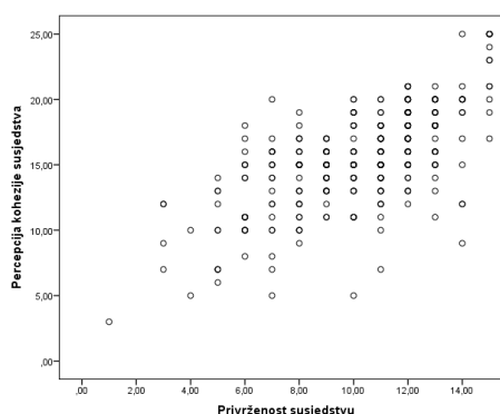
Prikaz 16.2. Dijagram raspršenja za varijable privrženosti susjedstvu i percepcije susjedske kohezije
