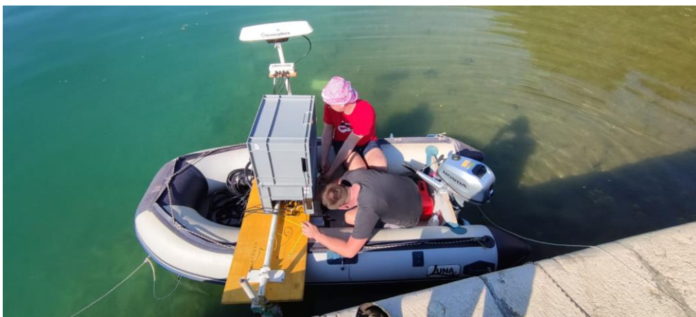
Slika 31. Gumenjak Luna s instaliranim integralnim mjernim sustavom
