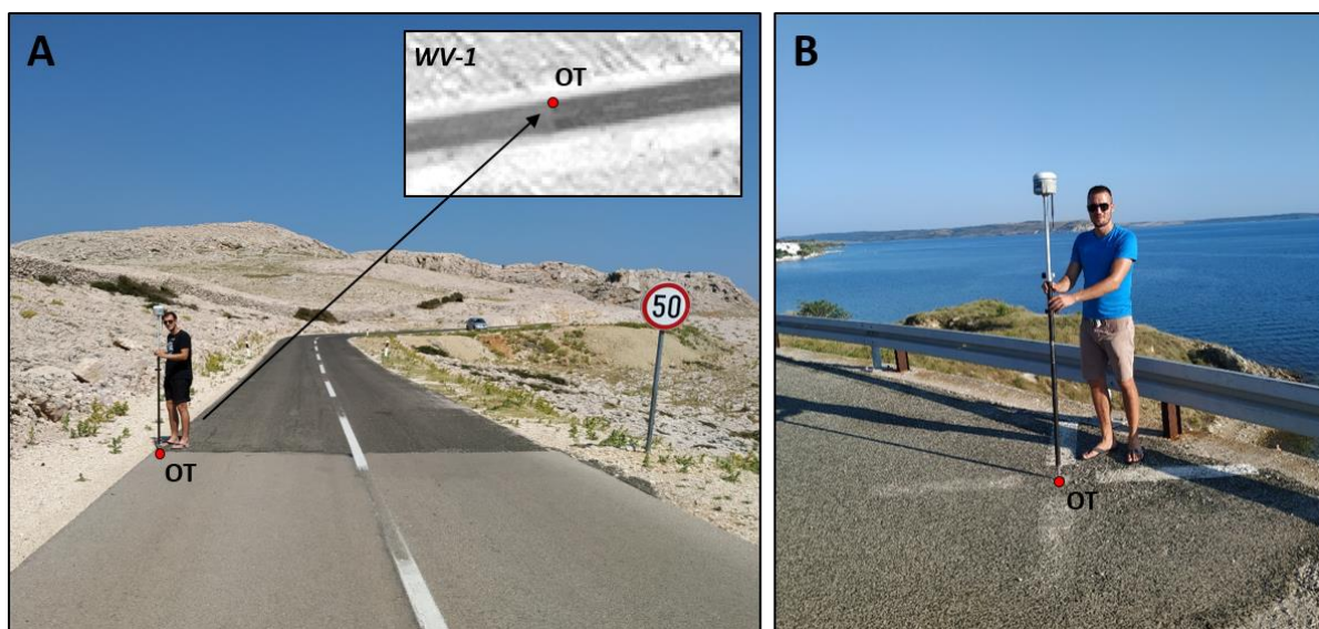
Slika 36. Terensko prikupljanje OT i KT sa Stonex S10 RTK GNSS-om (A – specifične oznake; B – postojeće geodetske oznake)
