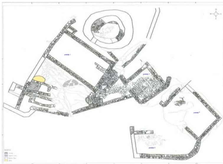
Slika 3. Tlocrt utvrde Nutjak (A. TABAK et al., 2010, 428).
