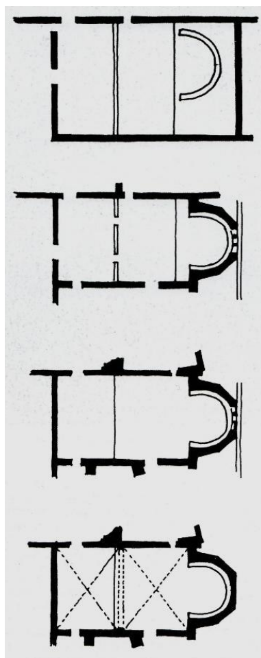
2. Zadar, Sv. Petar – razvojne faze katekumeneja od oratorija do sakristije (P. Vežić, 1990.)
