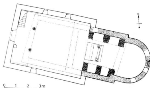
Slika 22. Tlocrt crkve Sv. Stjepana (S. S. GVOZDANOVIĆ, 2007., 199.)
