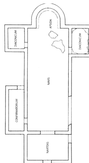
Slika 19. Tlocrt crkve Sv. Marije u Grohotama na Šolti (S. S. GVOZDANOVIĆ, 2007.)
