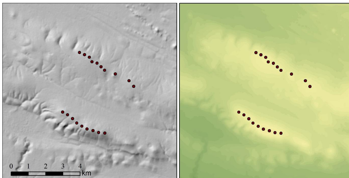
Slika 39. ALOS (AW3D30) DEM - sjenčani reljef (a) i hipsometrijska karta (b) na području VE „Danilo“
